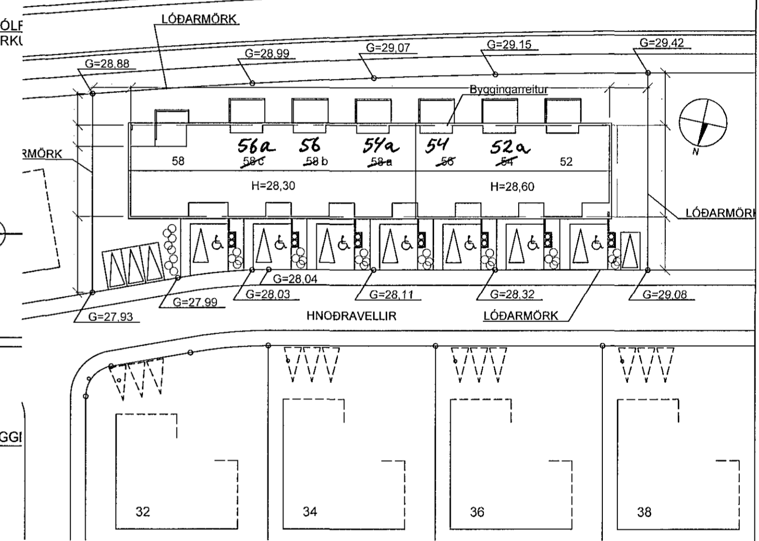
AFSTÖÐUMYND, 1:500
