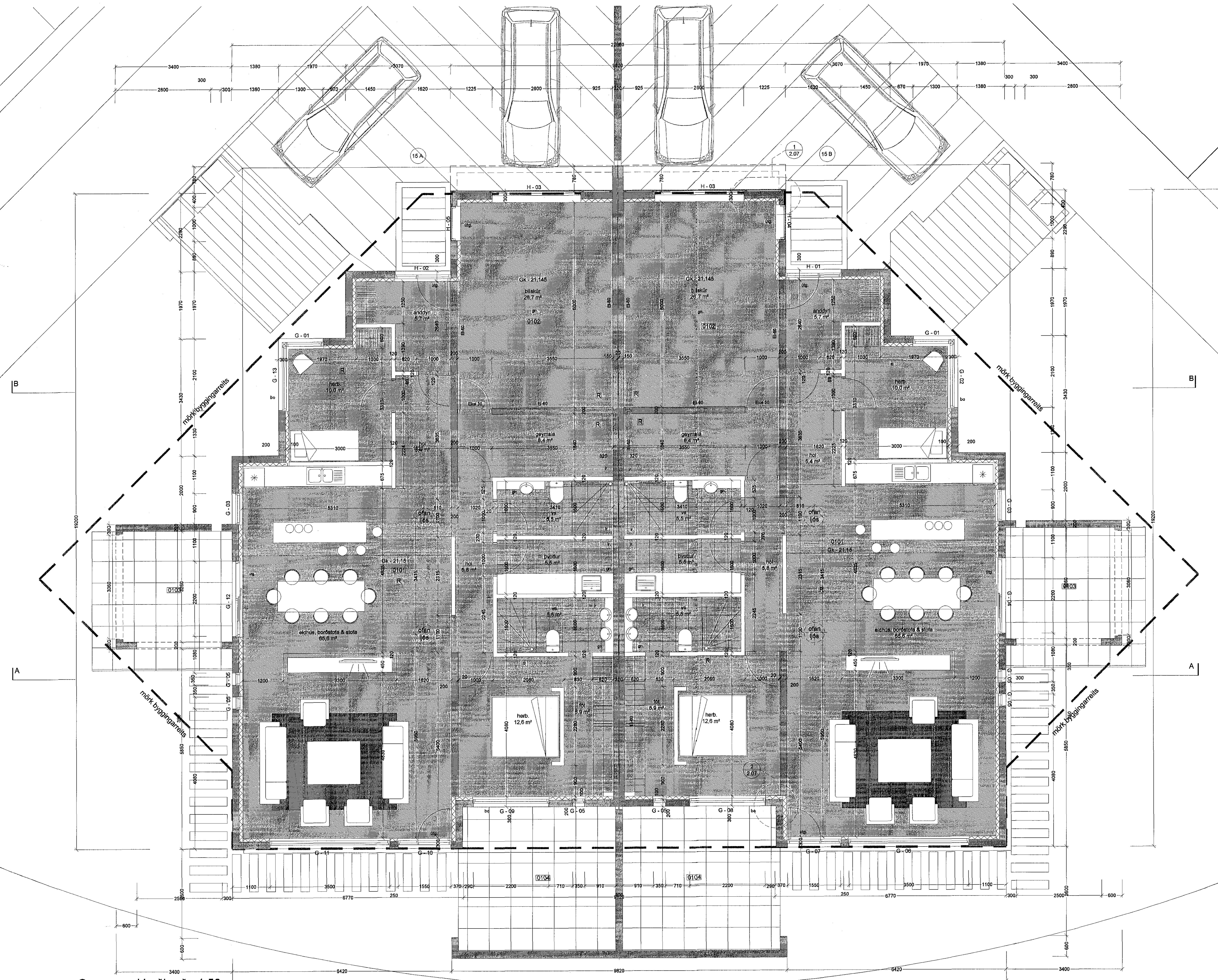
Grunnmynd jarðhæð - 1:50
