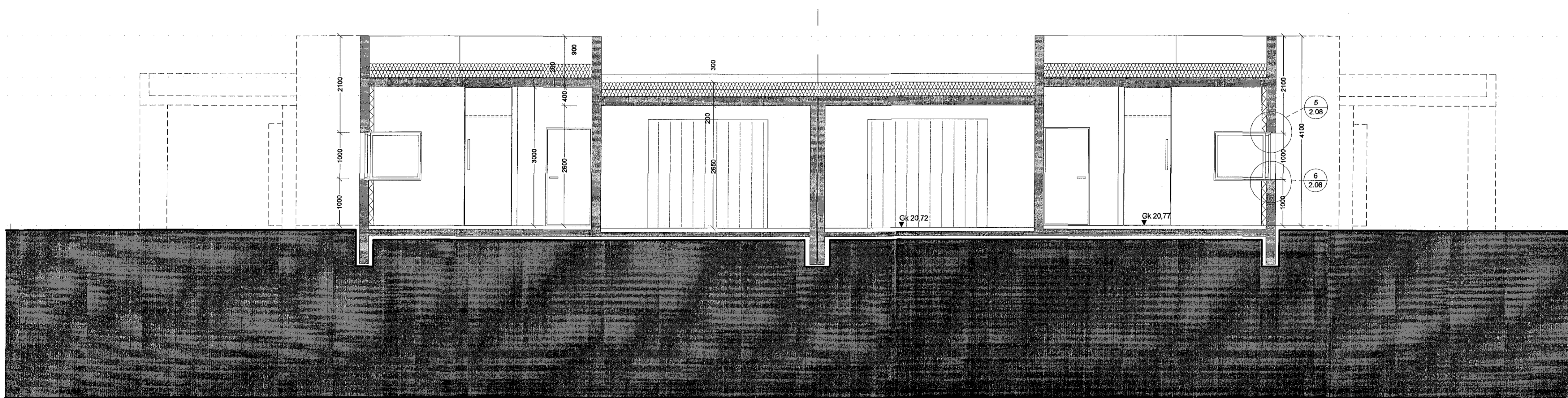
Sneiðing B-B / 1:50
