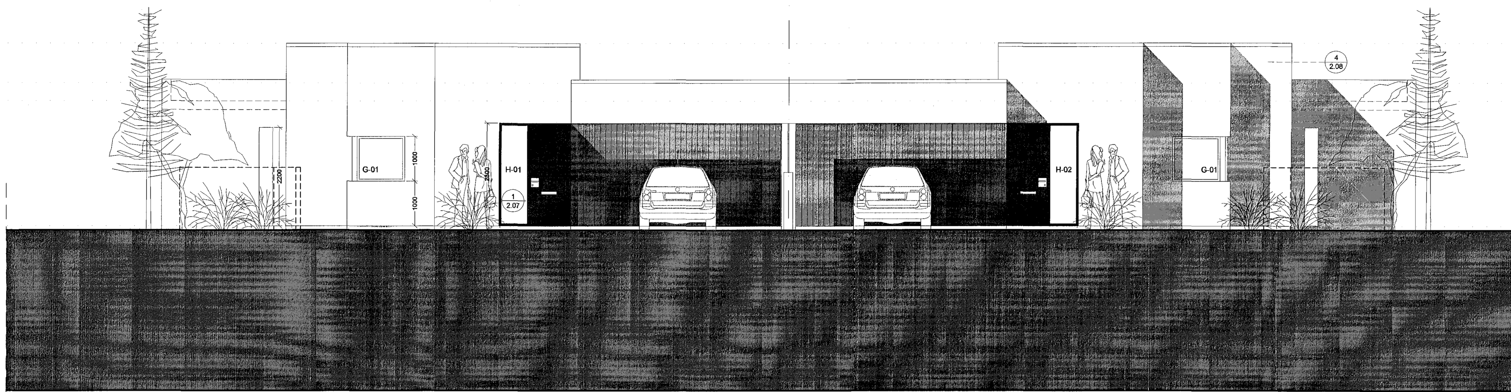
Útlit til suðausturs / 1:50
