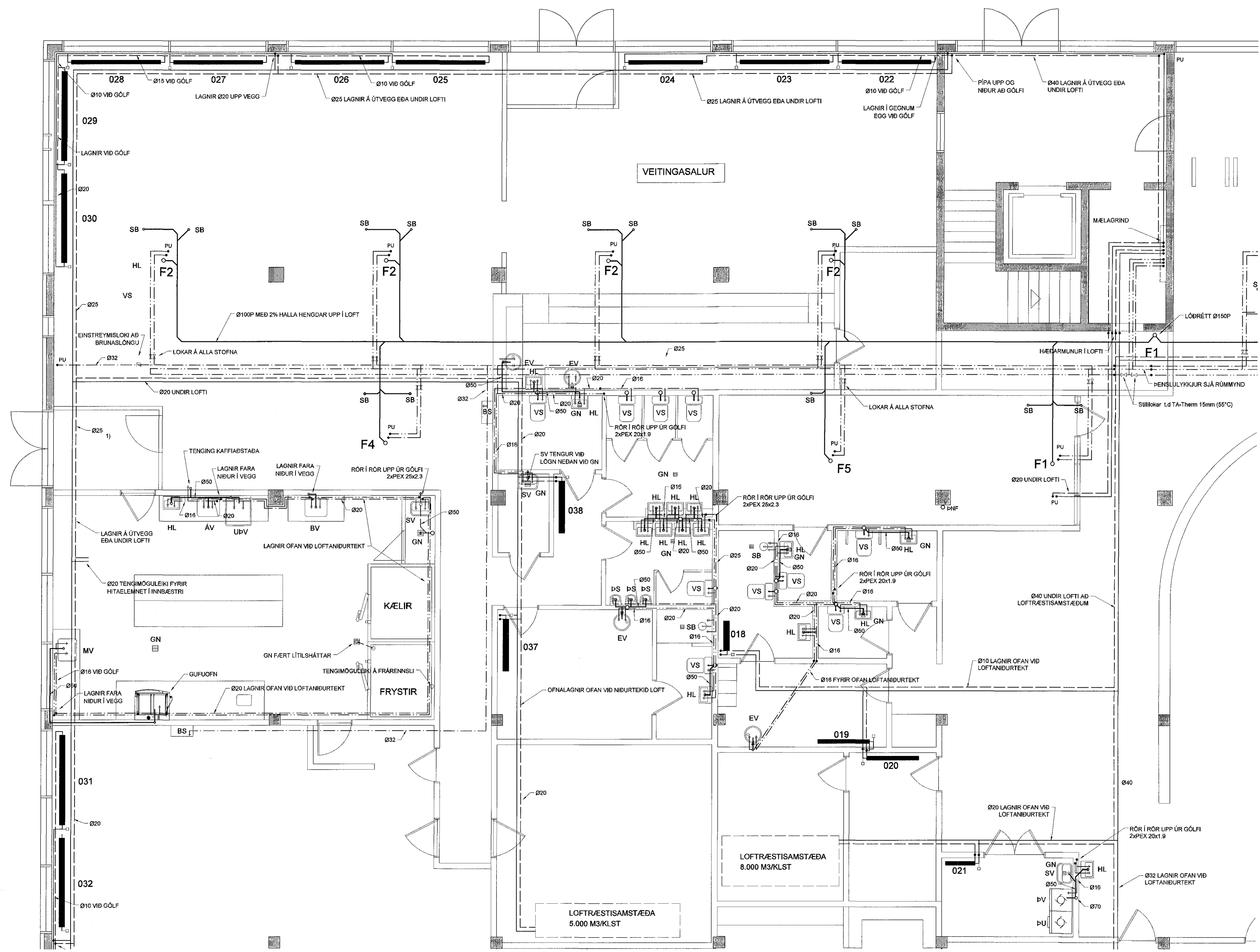
GRUNNMYND 1 1:50
