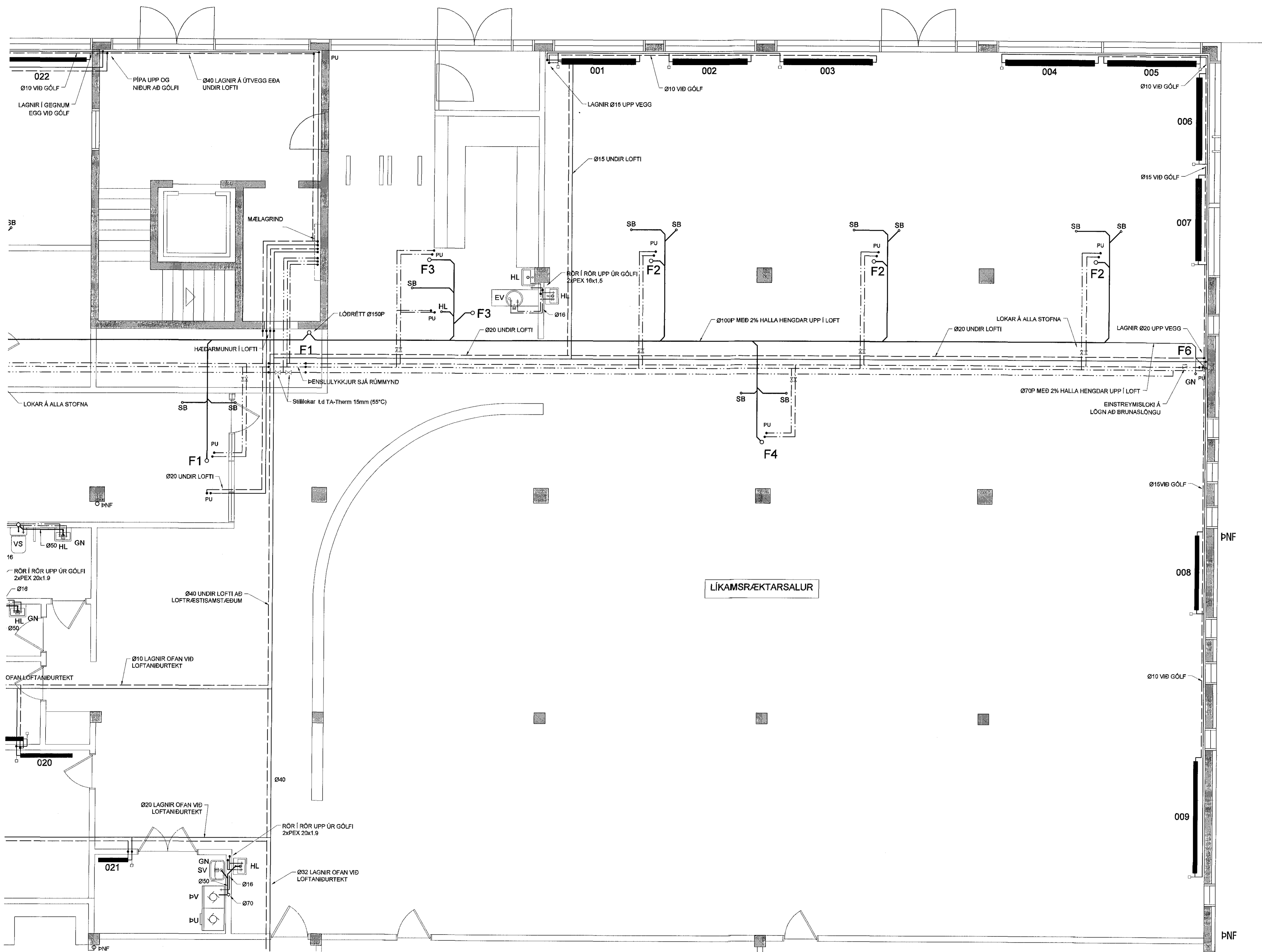
GRUNNMYND 3 1:50
