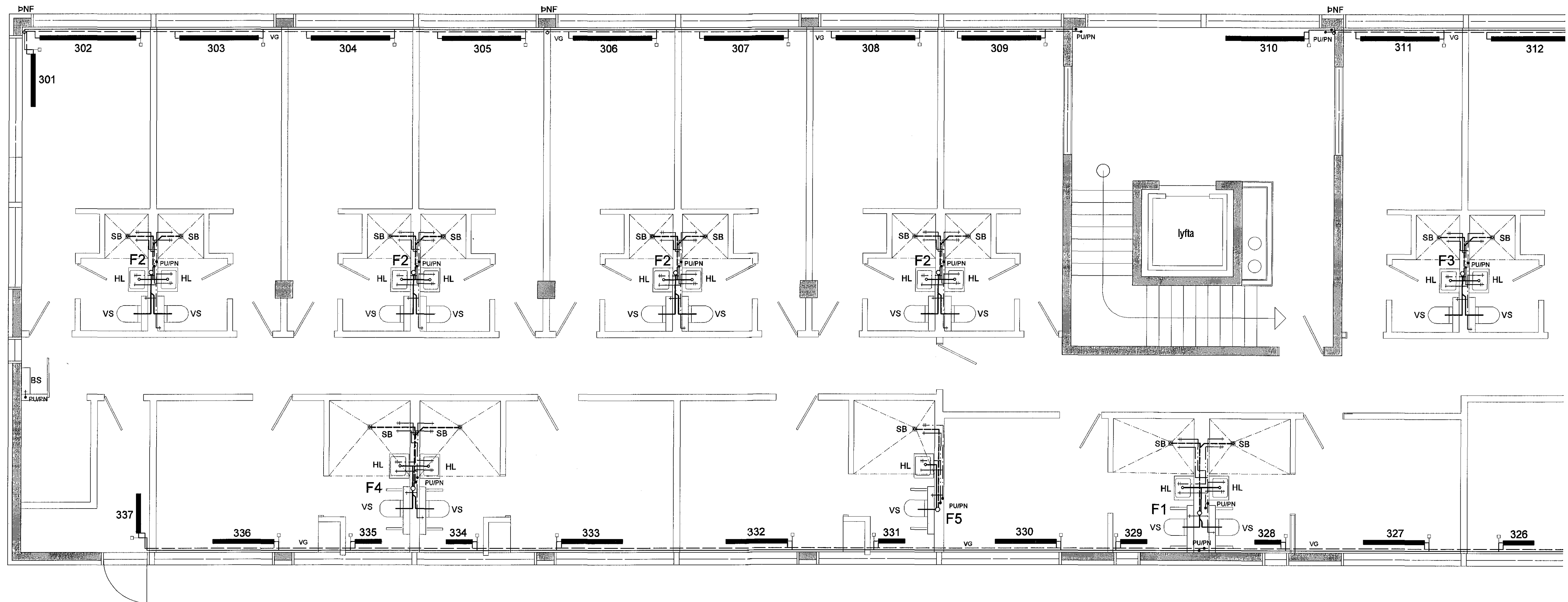
GRUNNMYND 3. HÆÐ - VESTURHLUTI 1:50
