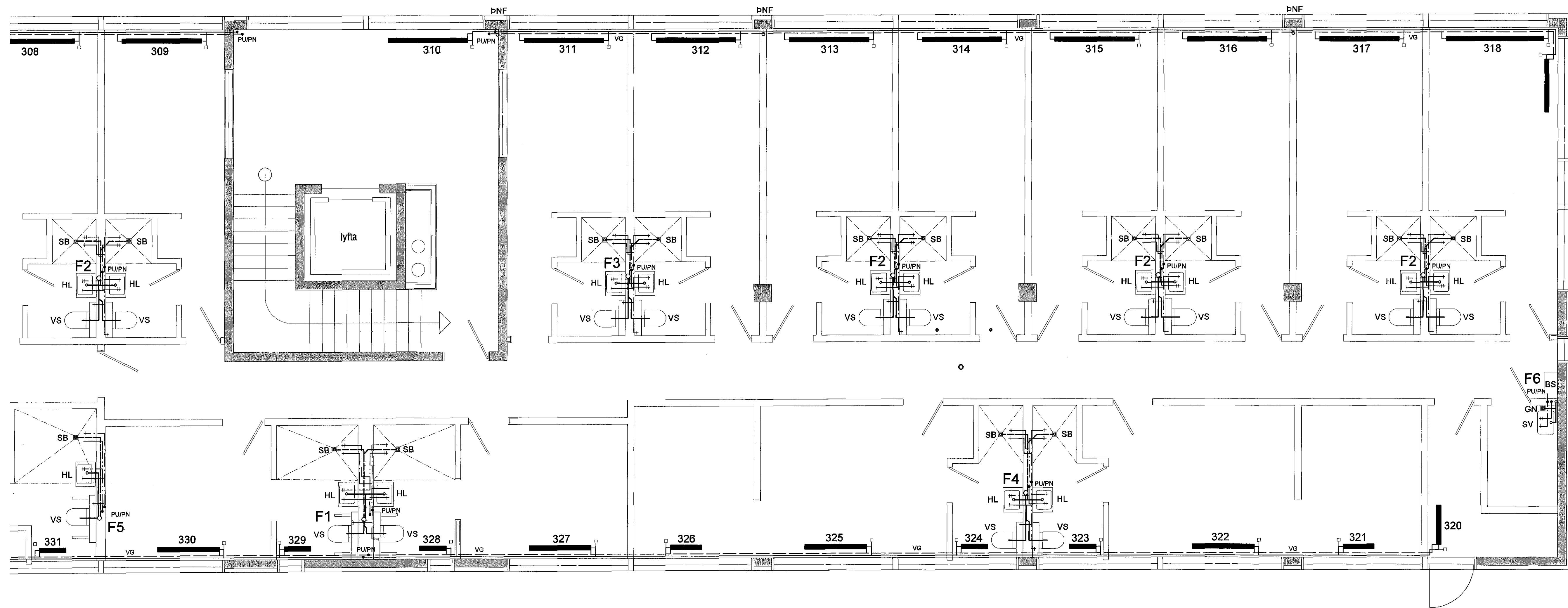
GRUNNMYND 3. HÆÐ - AUSTURHLUTI 1:50
