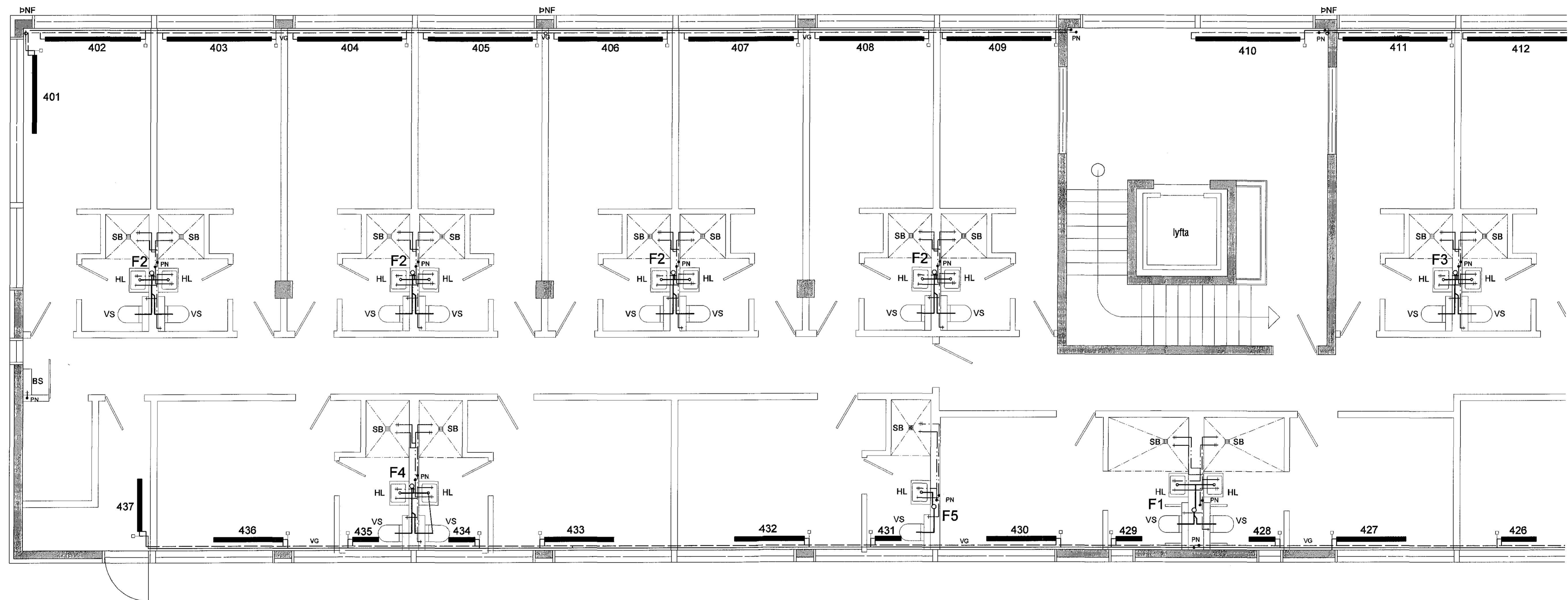
GRUNNMYND 4. HÆÐ - AUSTURHLUTI 1:50
