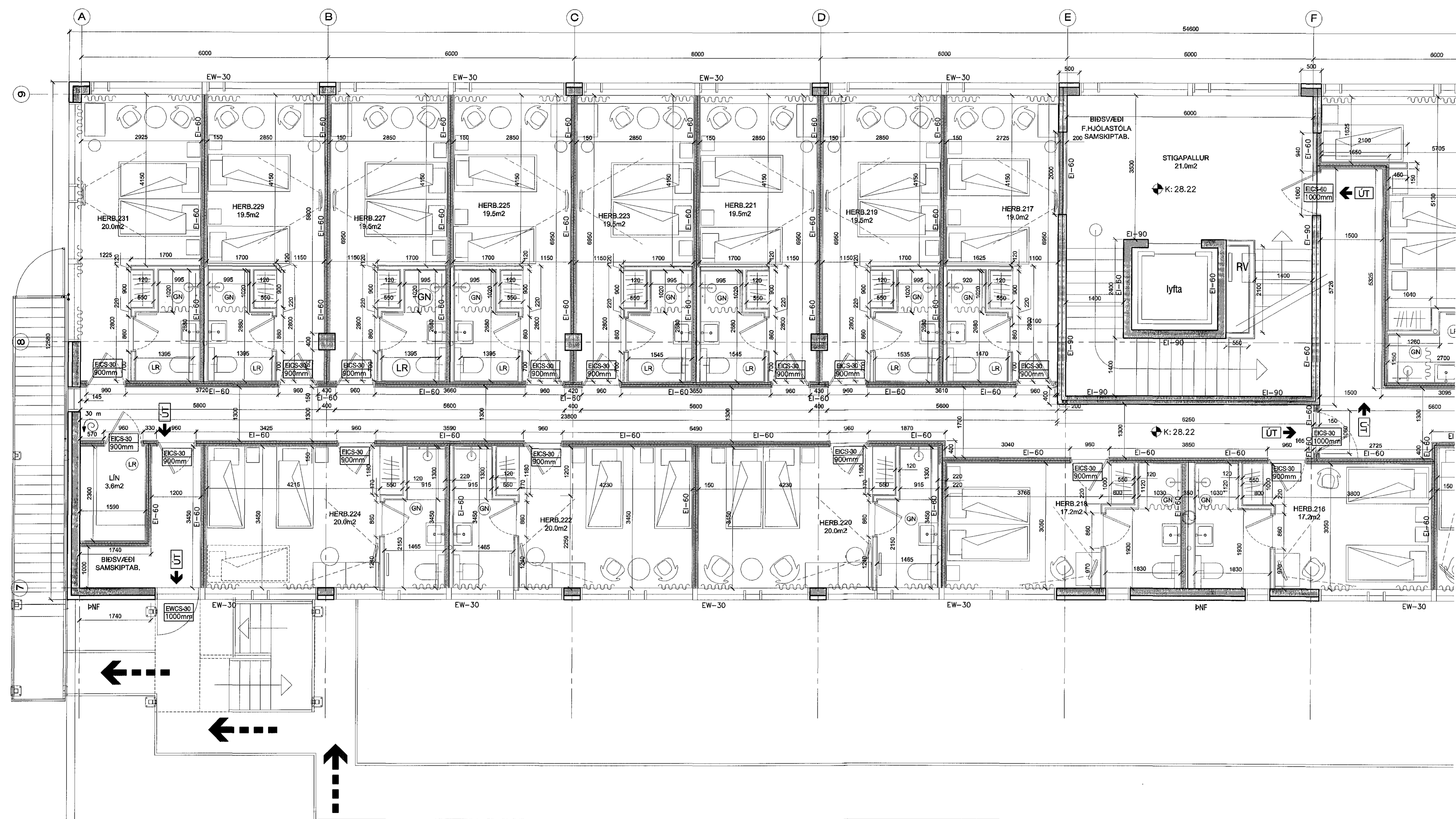
Grunnmynd 2.hæð - vestur mkv. 1:50
