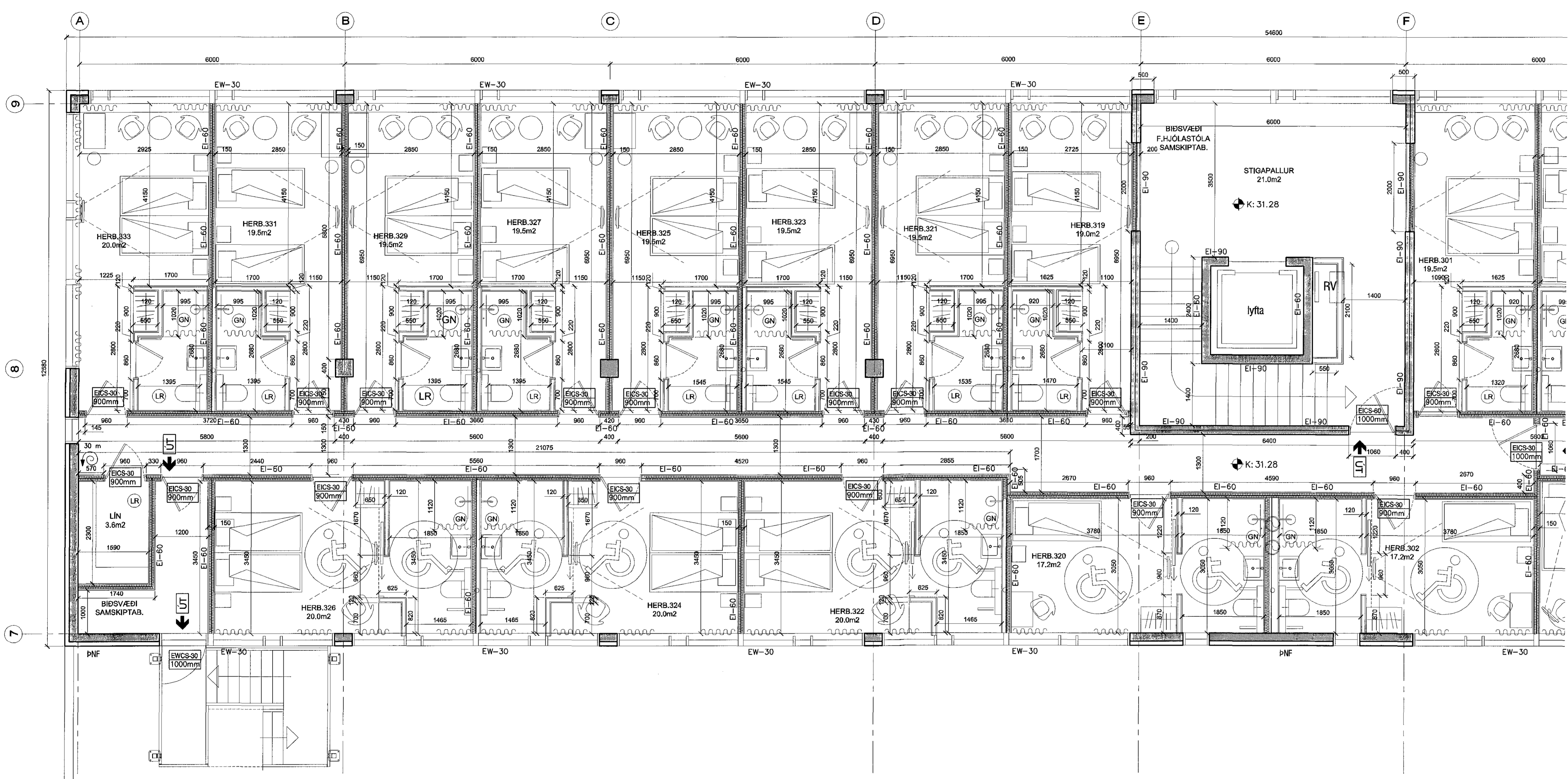
Grunnmynd 3.hæð - vestur mkv. 1:50
