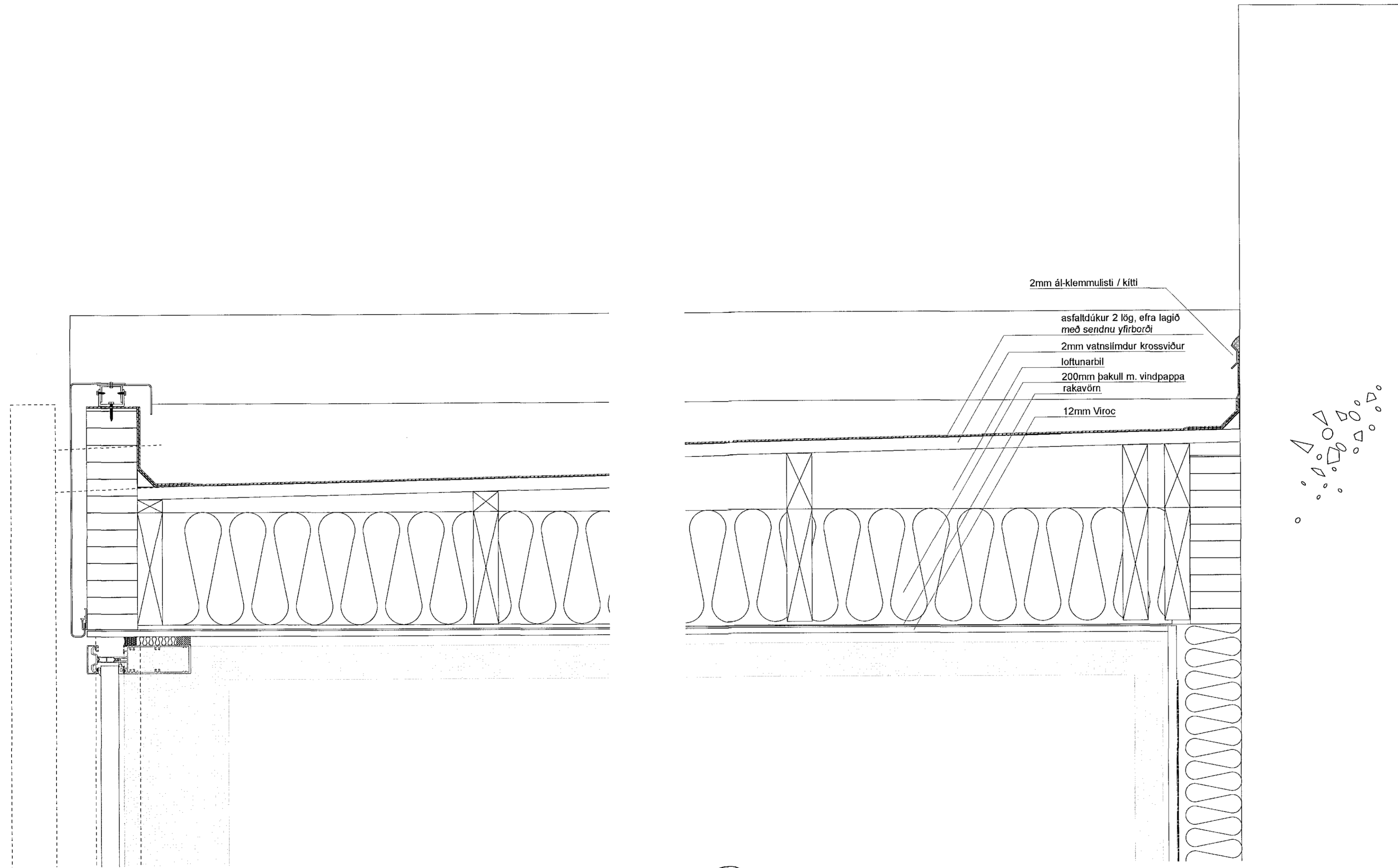
2 A-402 LÓDRÉTT DEILI mkv. 1:5
