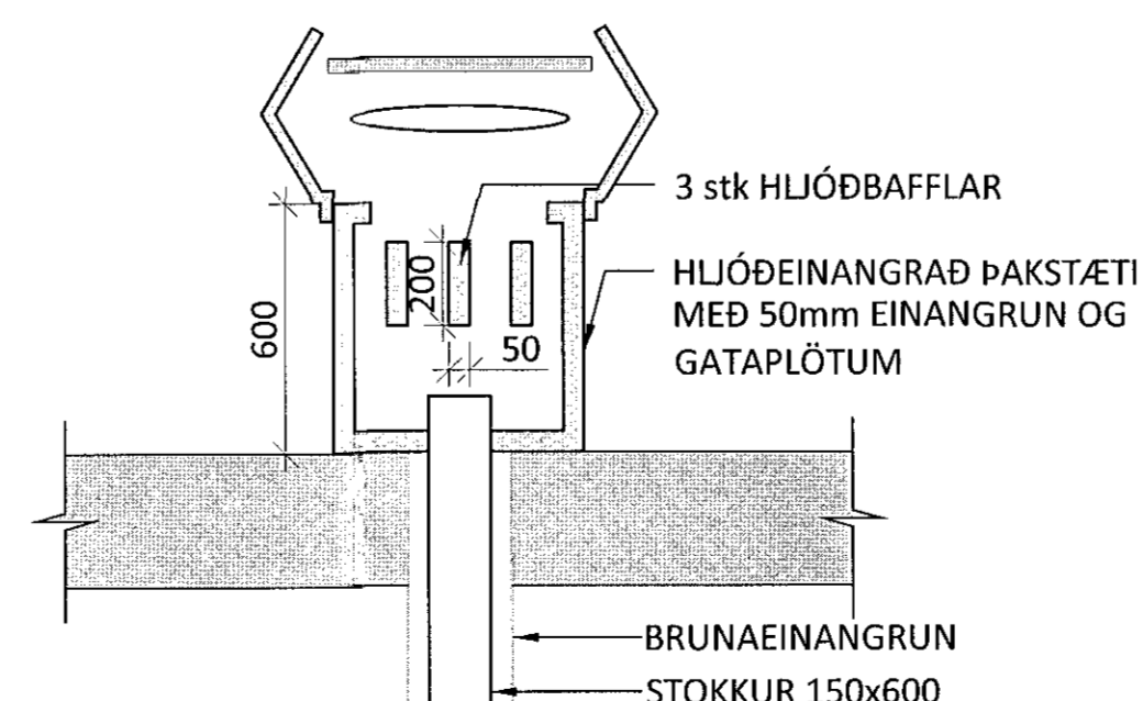
ÞAKBLÁSARI 8ÚB1 M.1:20
