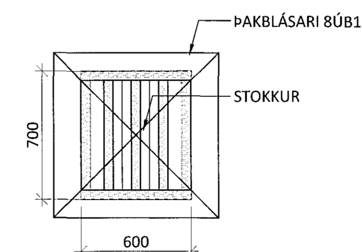
UNDIRSTADA ÞAKBLÁSARA - SÉÐ AÐ OFAN M.1:20
