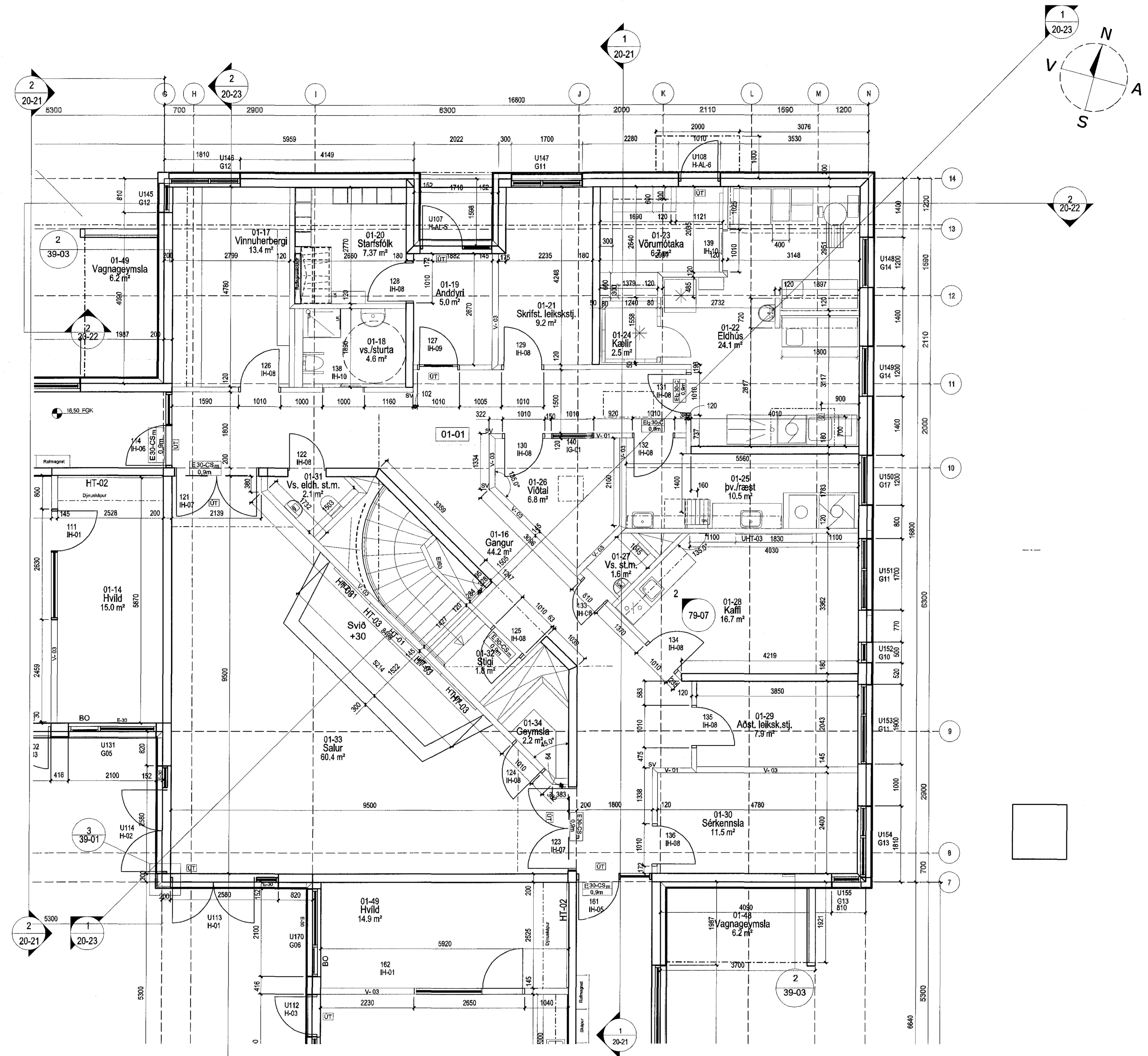
2 Grunnmynd 1. hæð 20-03 1:50
