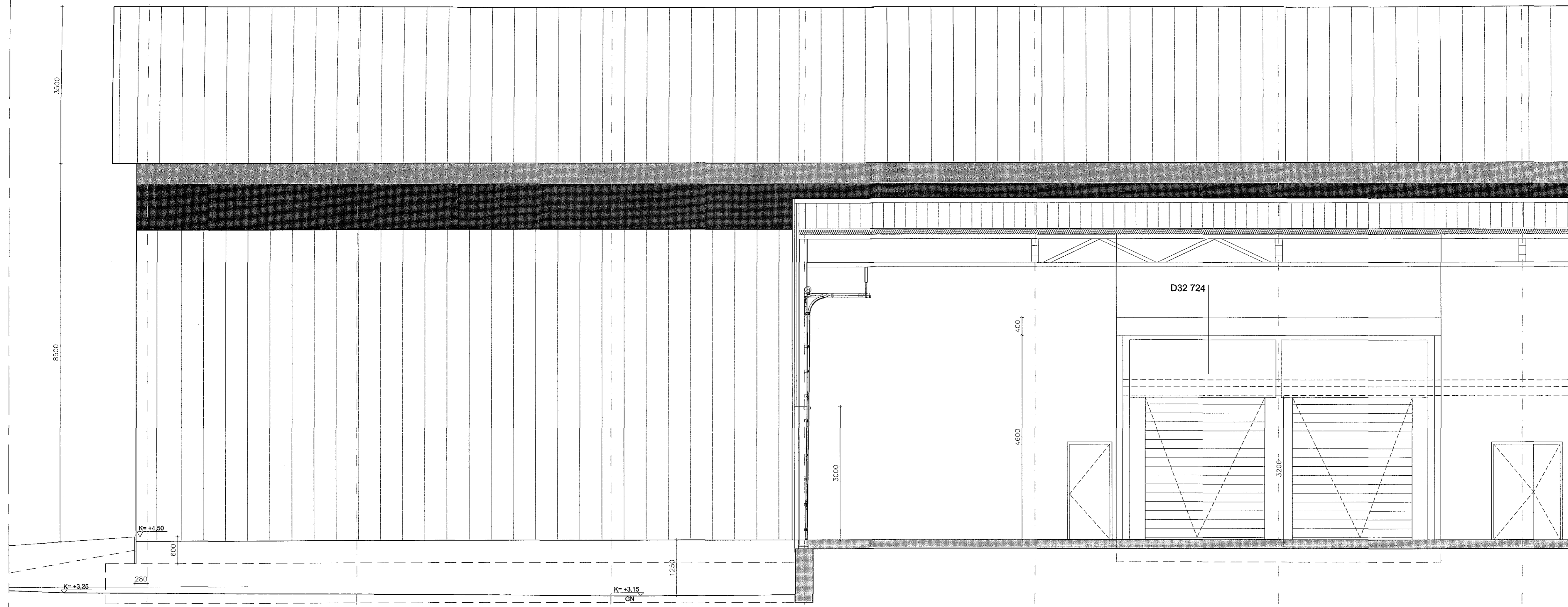
1000 frá skákli SNID B-B MKV.1:50
