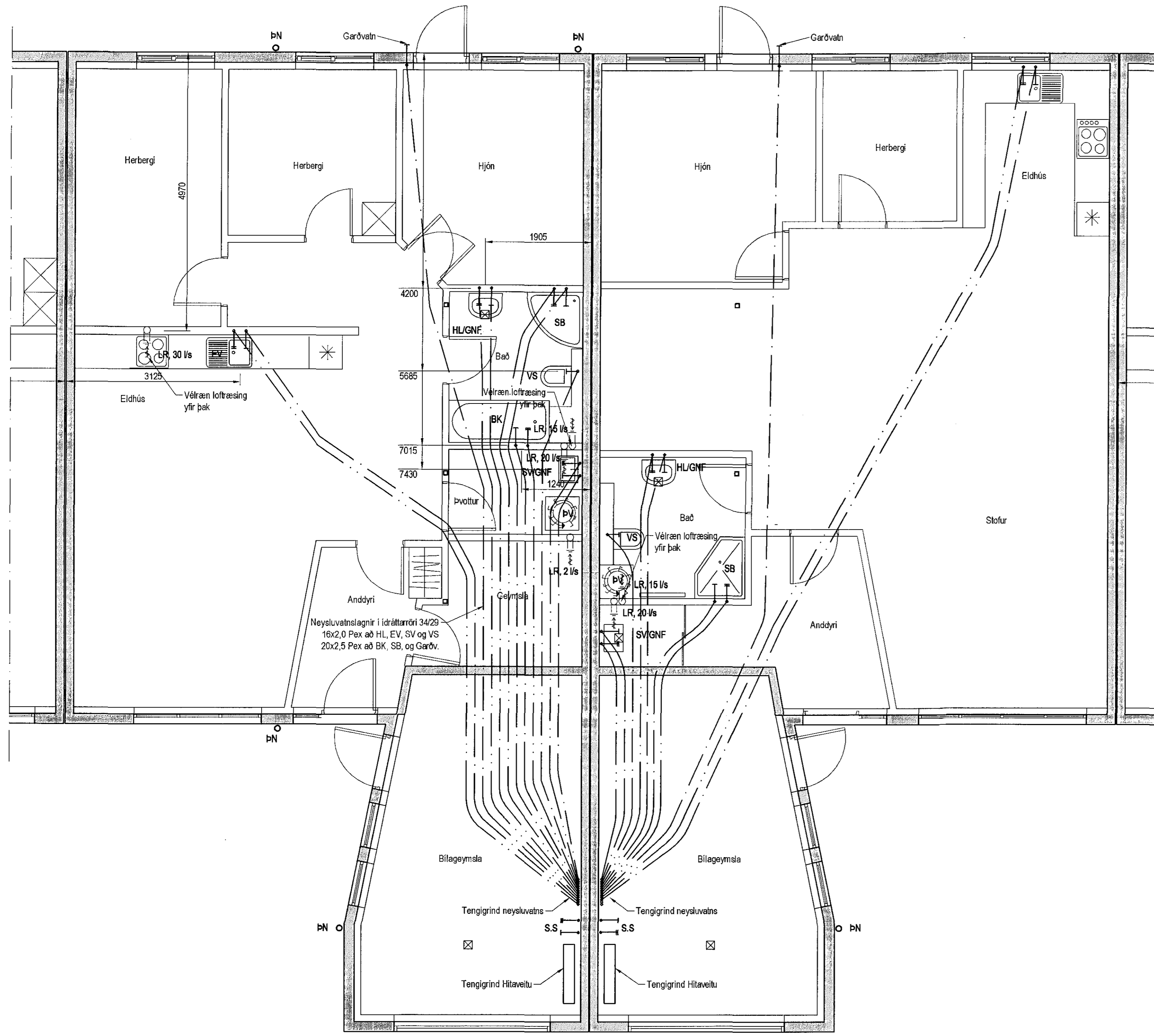
Neysluvatnslagnir 1. hæð, 1:50
