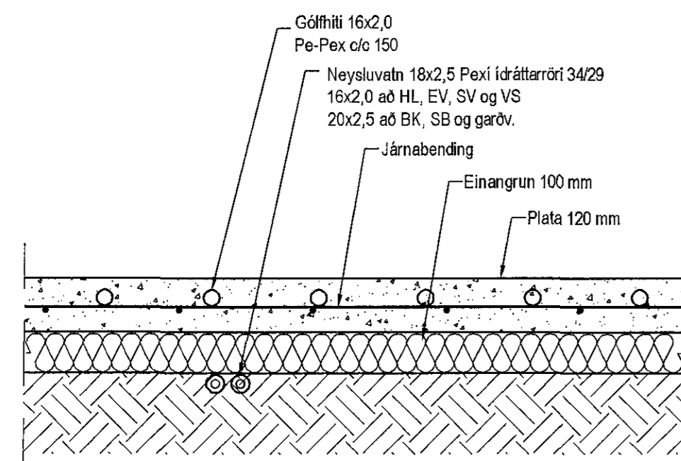
Hita- og vatnslagnir, Sníð í botnplötu bilageymstu, 1:10
