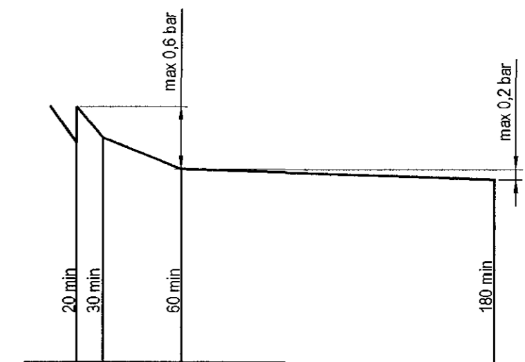
Þrýstiprófun á neysluvatnslagnum línurit
