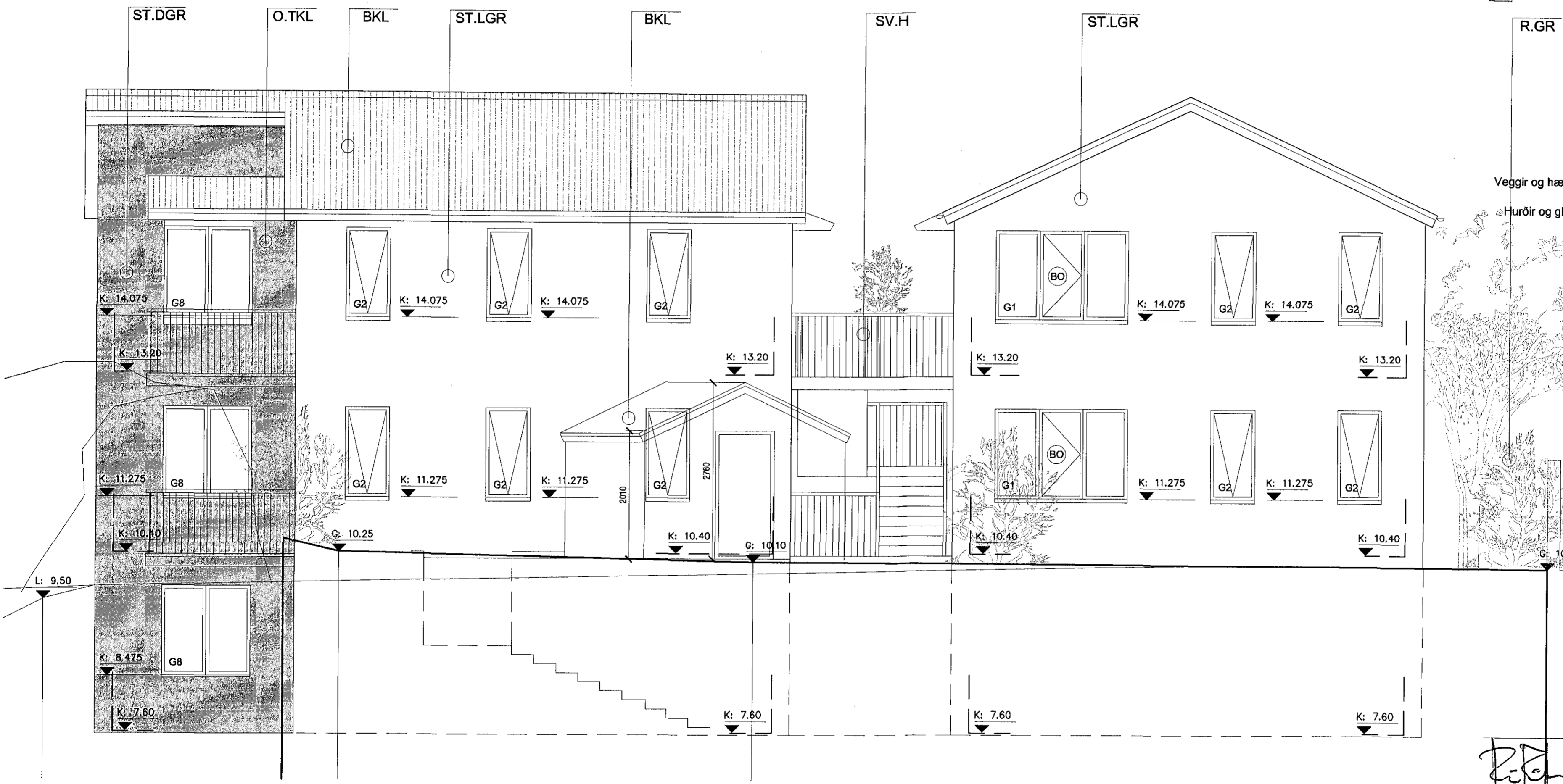
Ásýnd norð-austur mkv. 1:50
