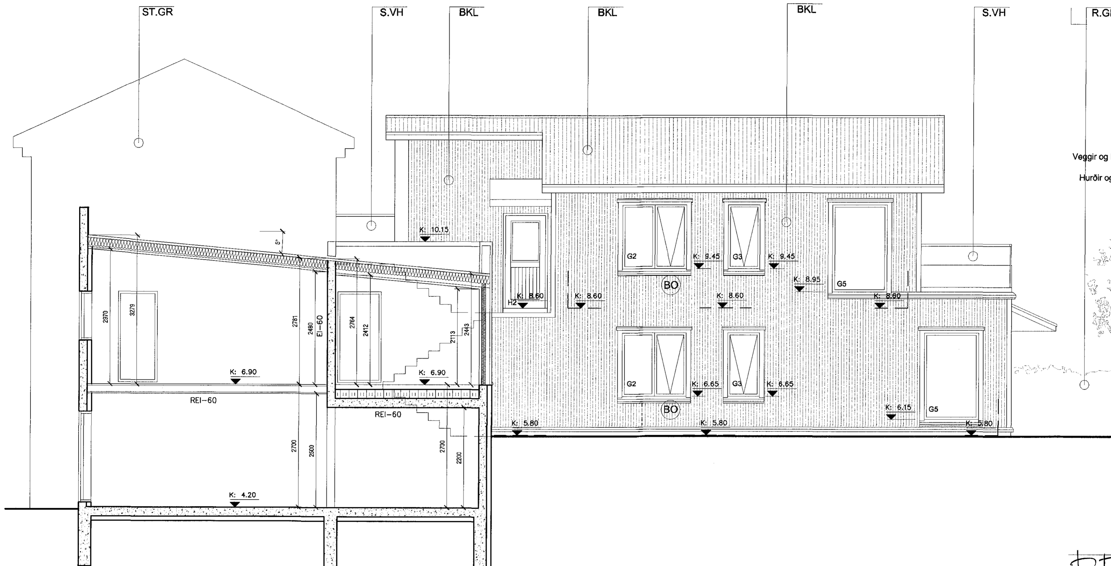
Sneiðing B-B / Ásýnd suð-austur mkv. 1:50
