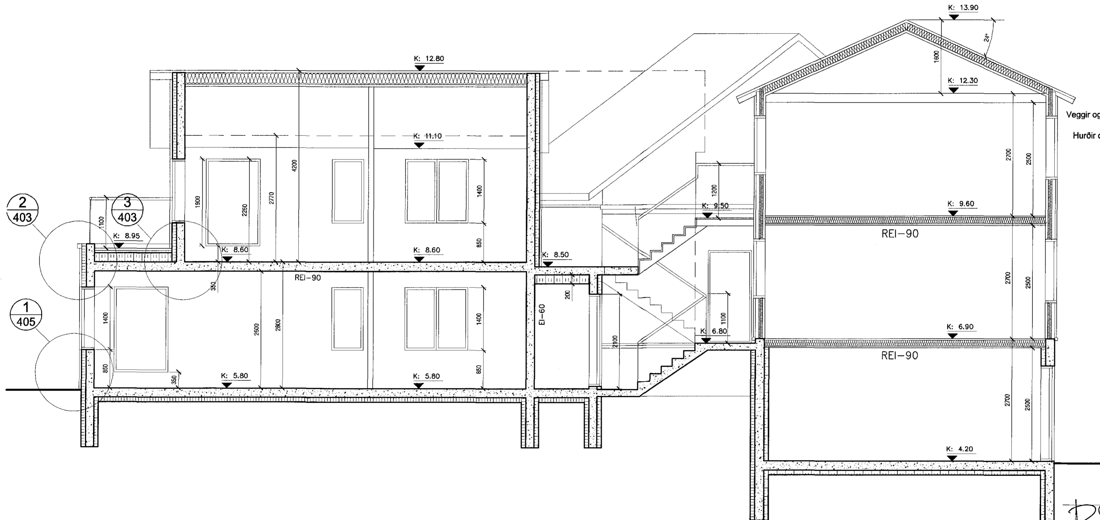
Sneiðing A-A mkv. 1:50
