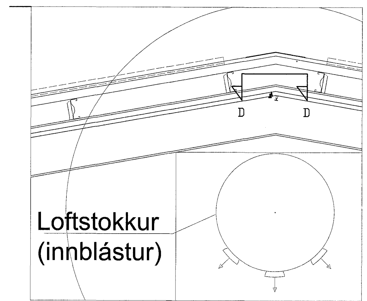
Snið C Mkv. 1:20.
