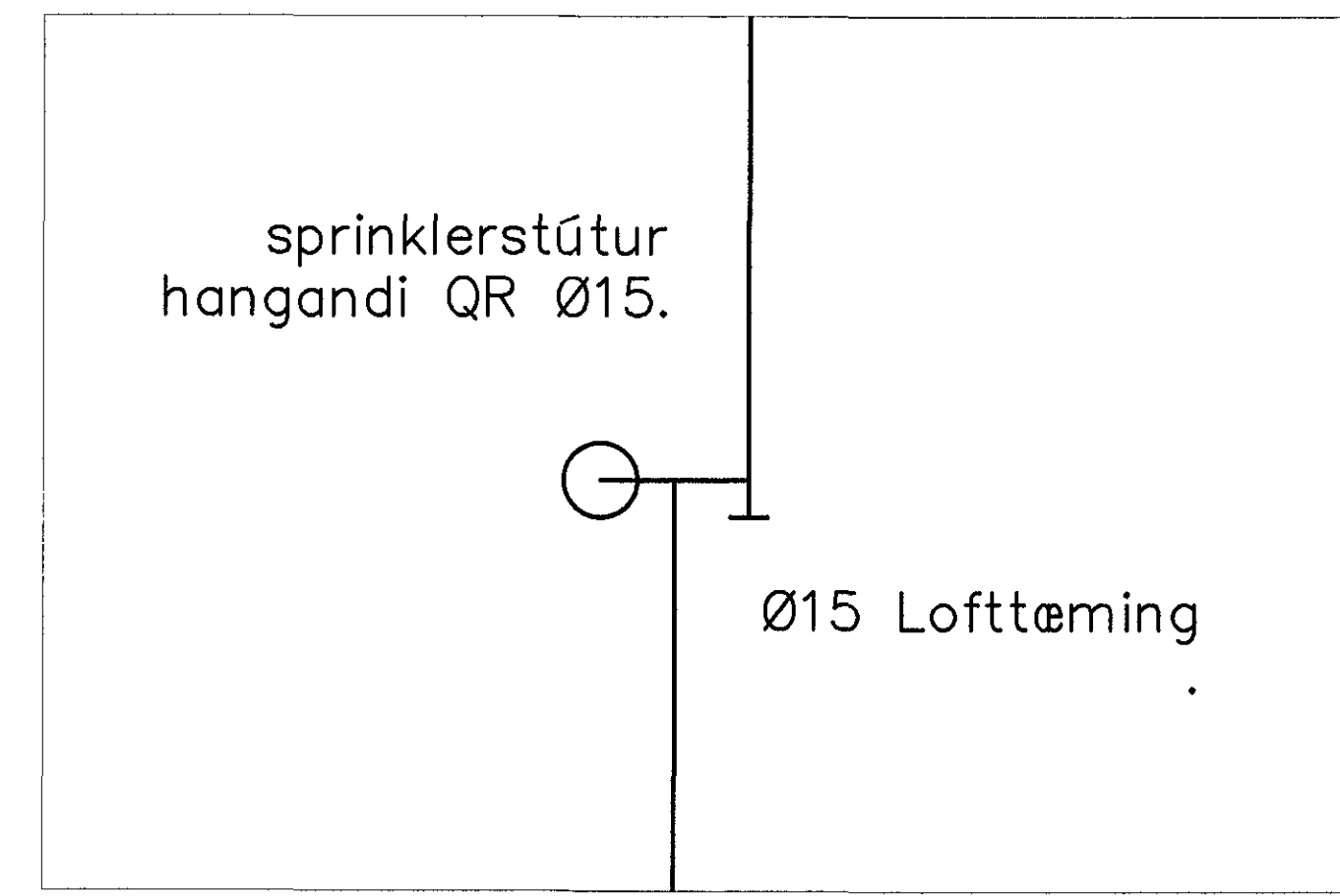
Snið D Mkv. 1:10.
