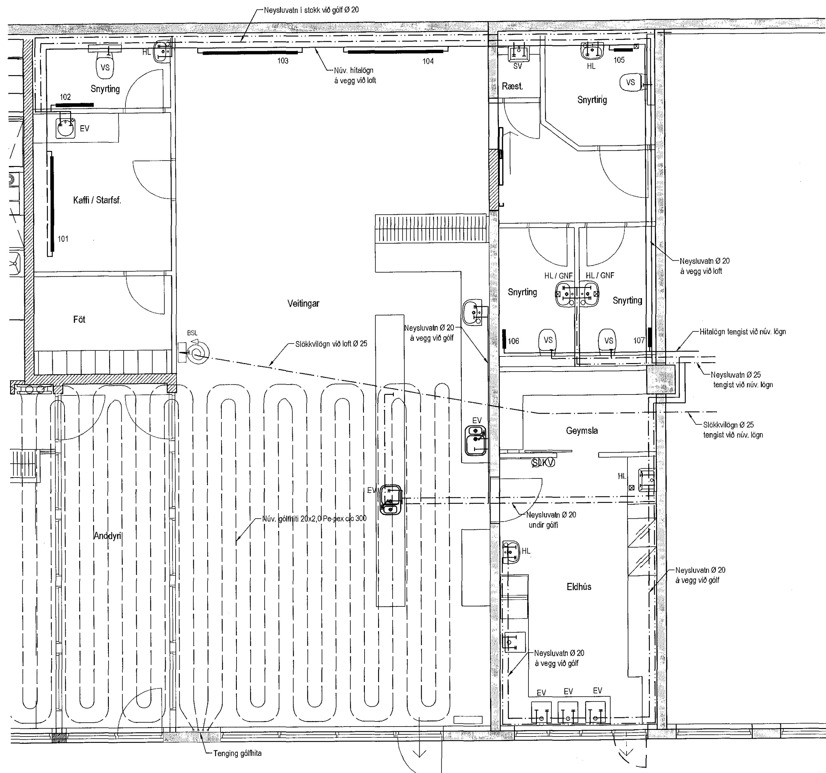
Hita- og Neysluvatnslagnir rými 01-03, Grunnmynd, 1:50
