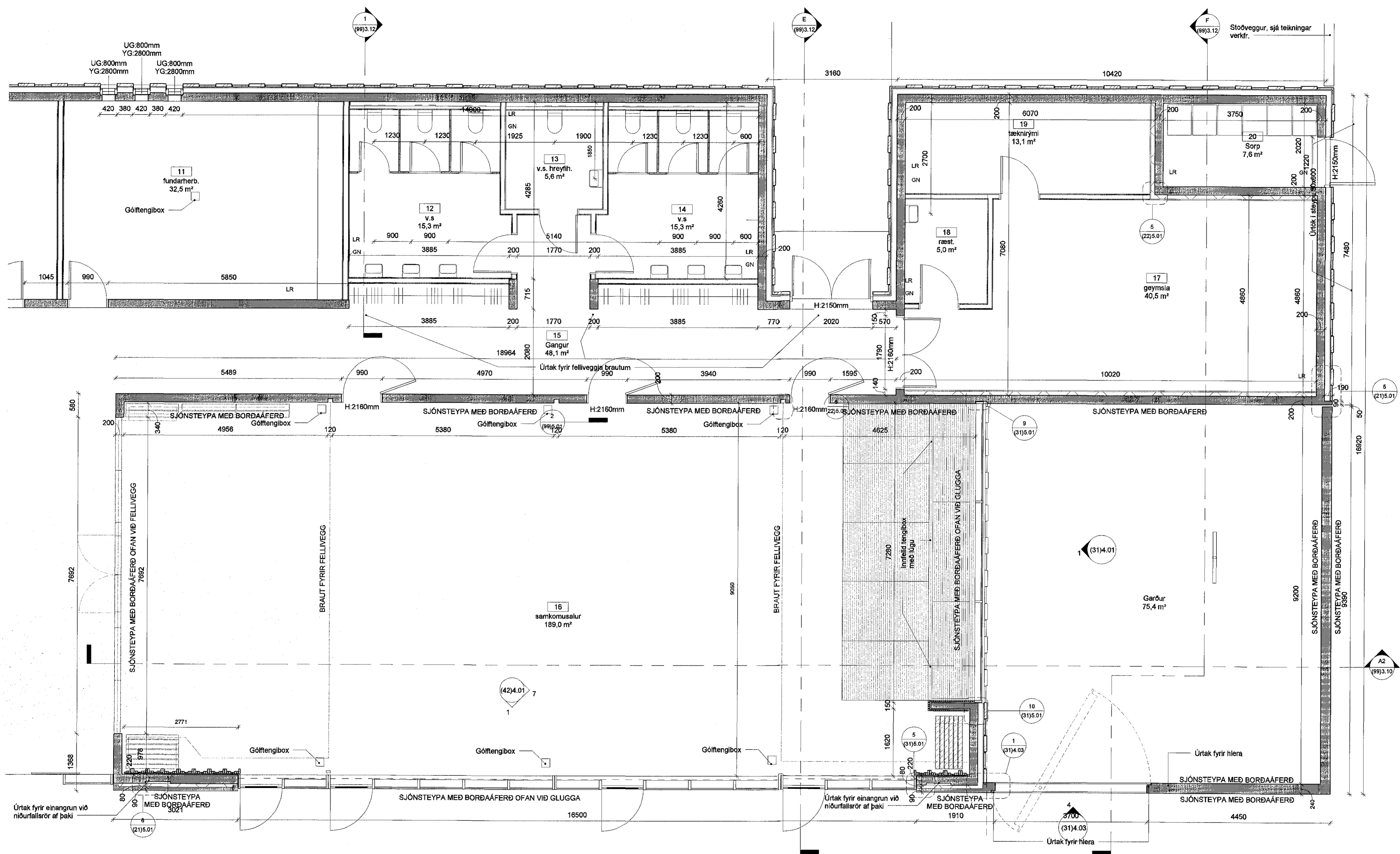
1 (21) Steyputeikning 2 af 2 1 : 50
