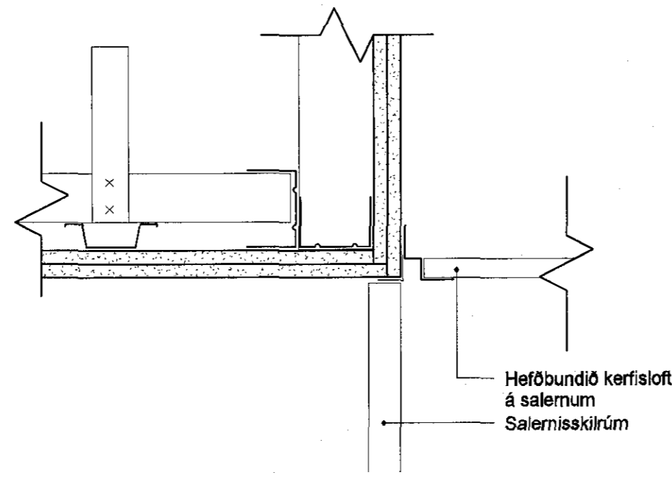
2 (45) LÓ - Fast loft yfir salernum 1:5
