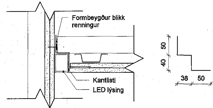
1 (45) LÓ - Lýsing á salernum 1:5
