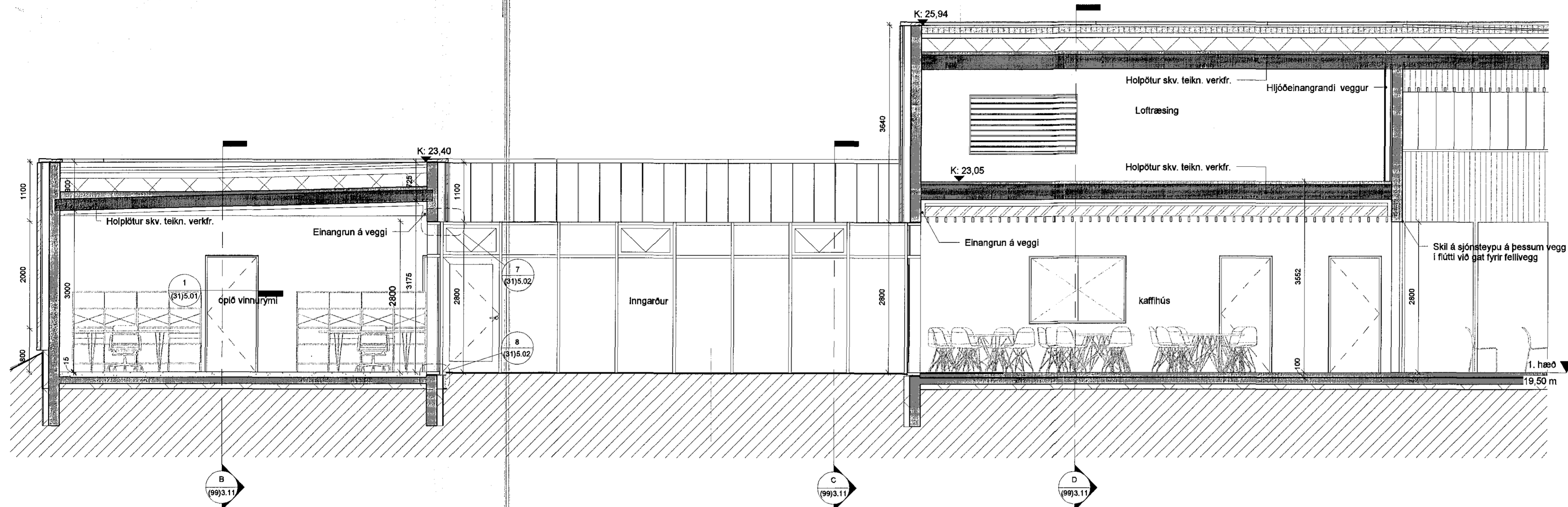
A (99) Snið A - A, HLUÐI 1 1 : 50
