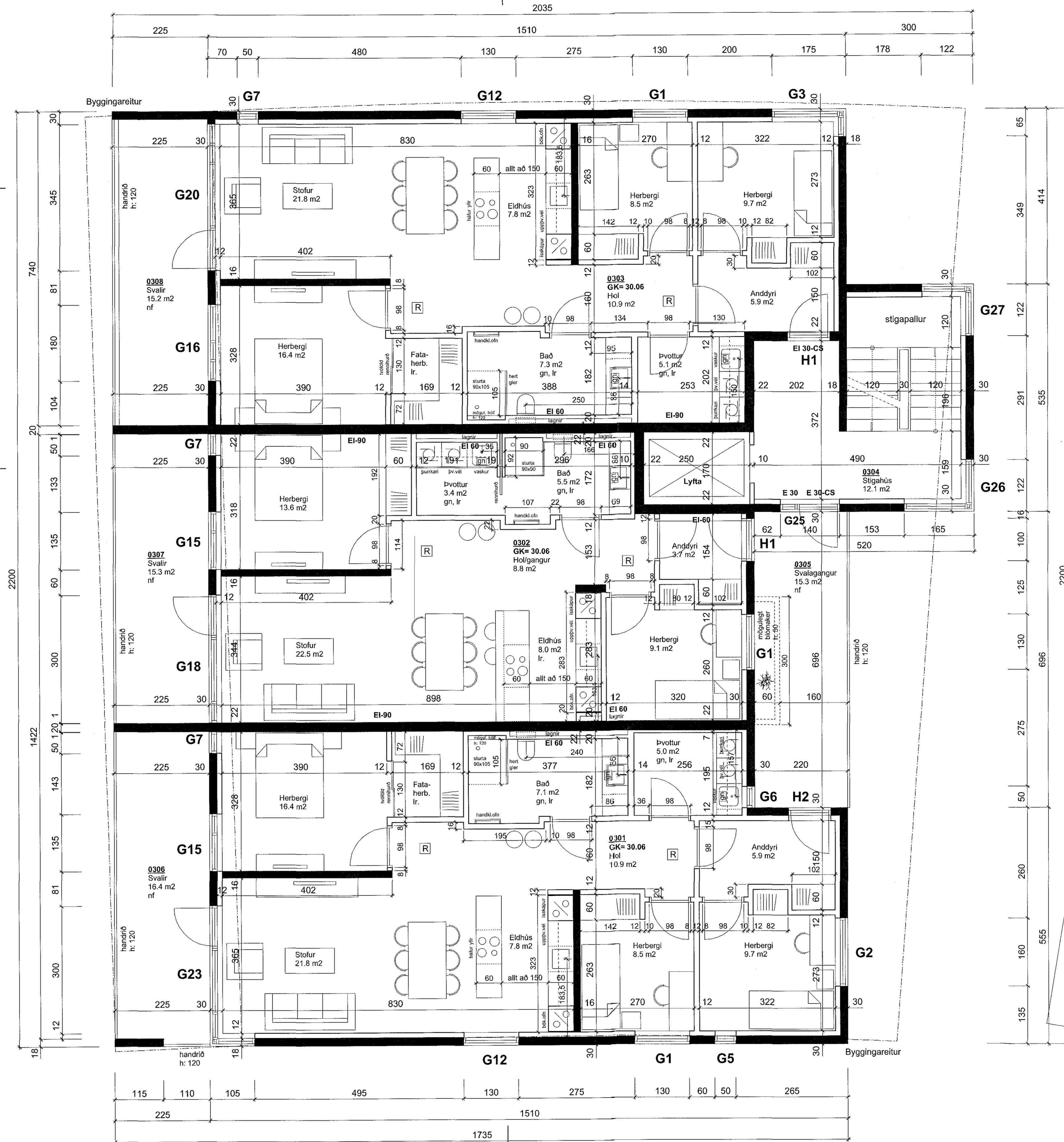
GRUNNMYND 3.hæðar
