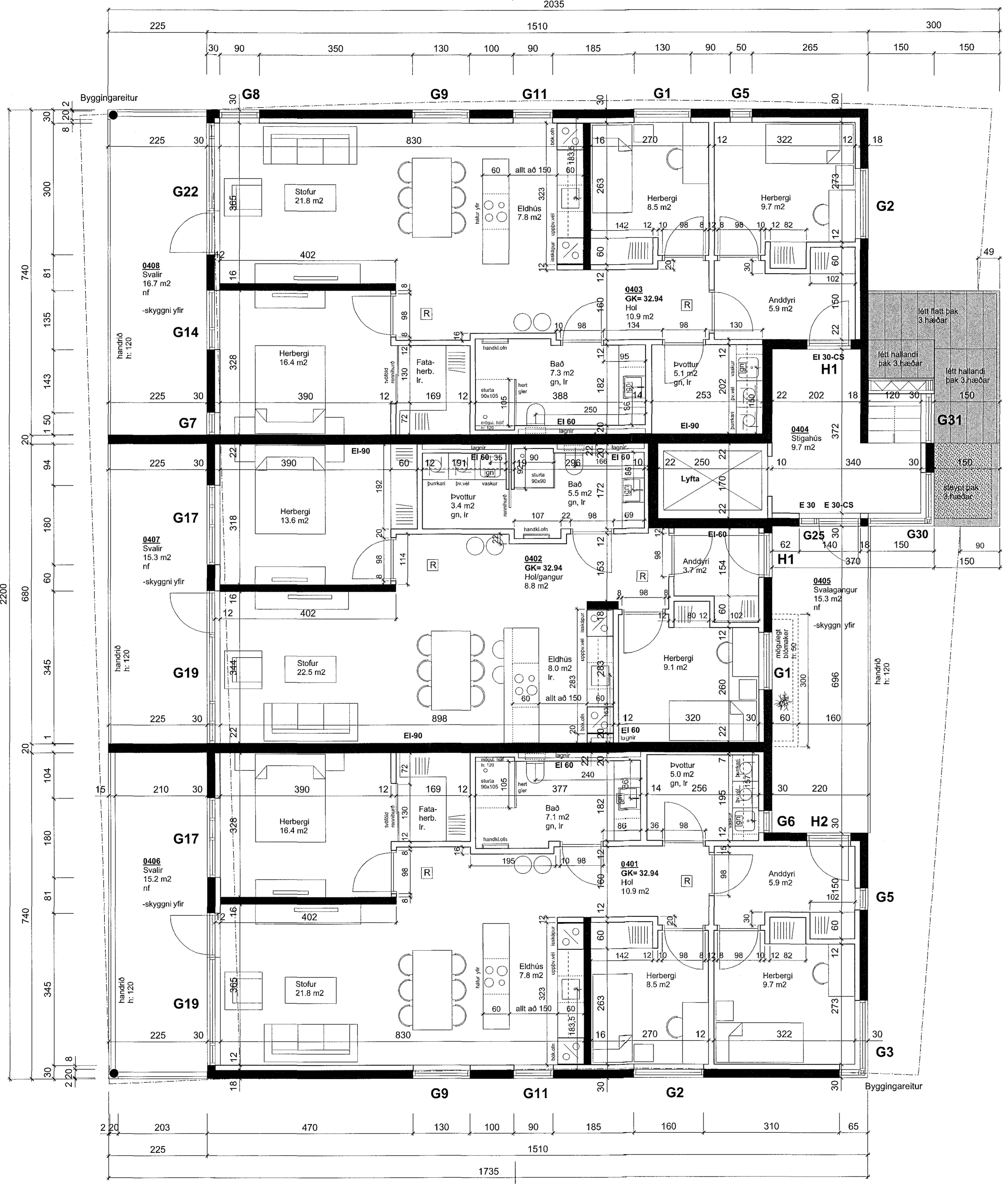
GRUNNMYND 4.hæðar
