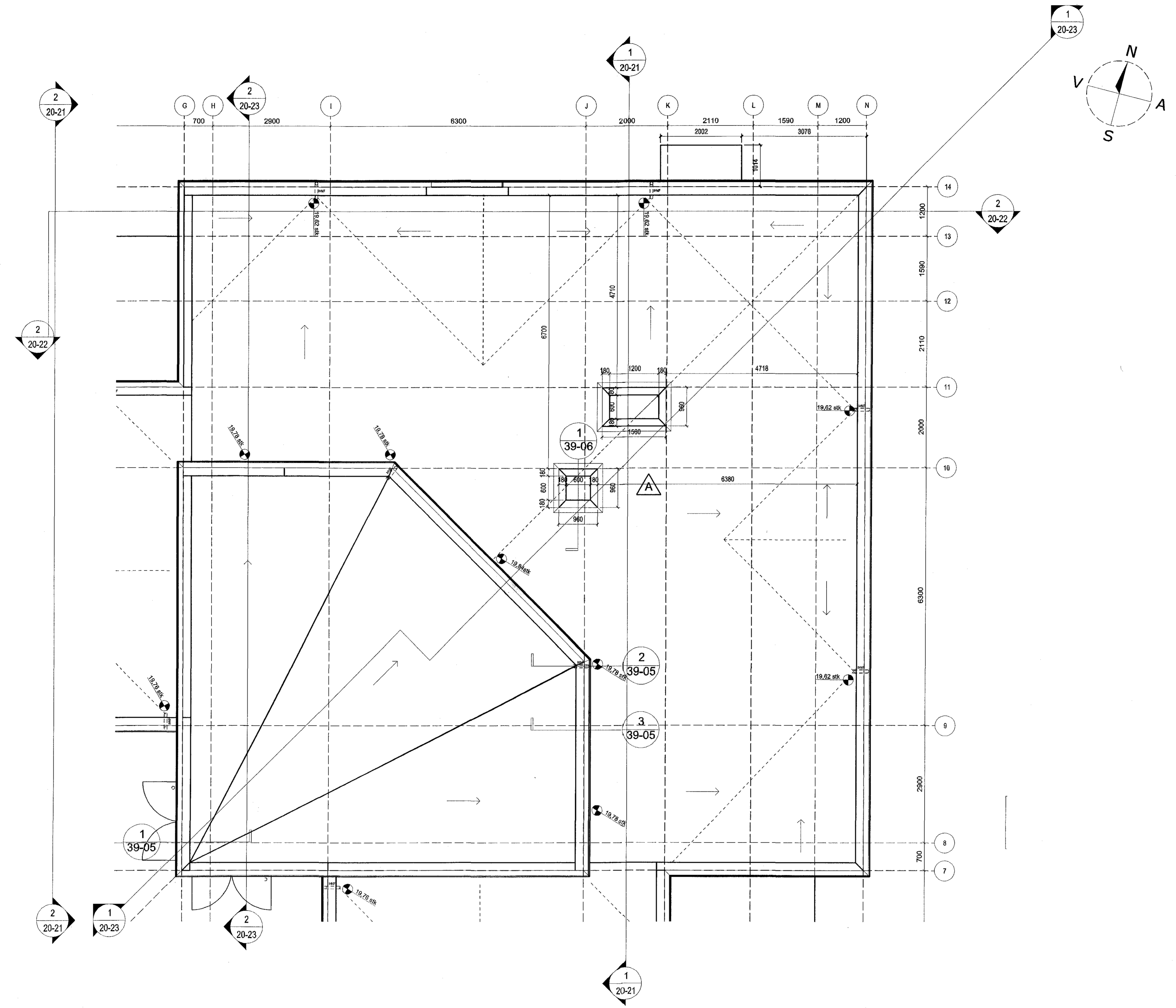
1 Þakmynd 20-06 / 1:50
