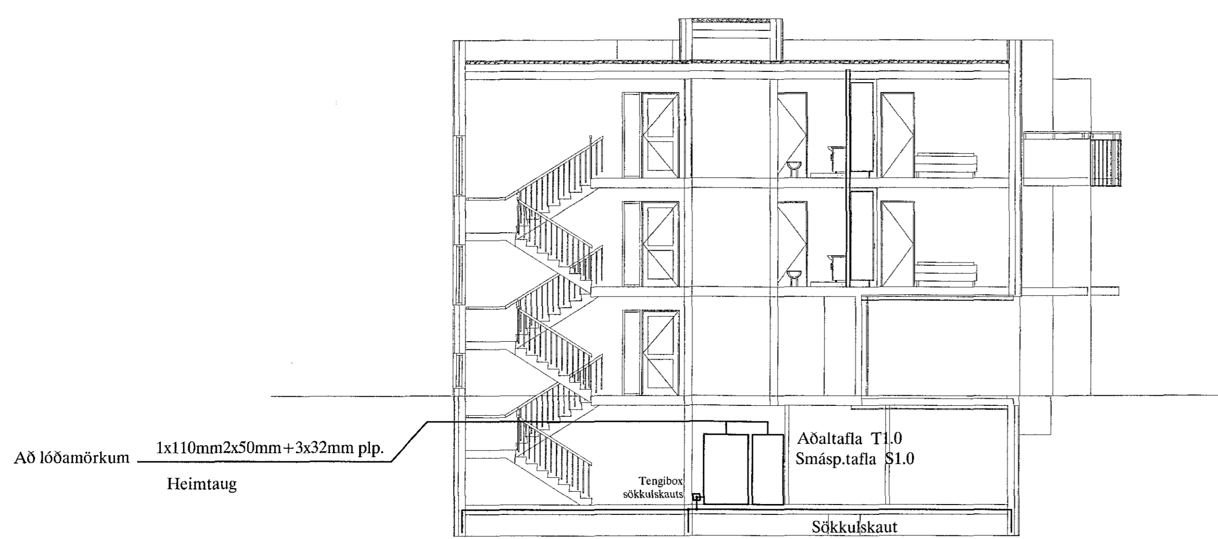
SNIÐ Í INNTAK M. 1:100
