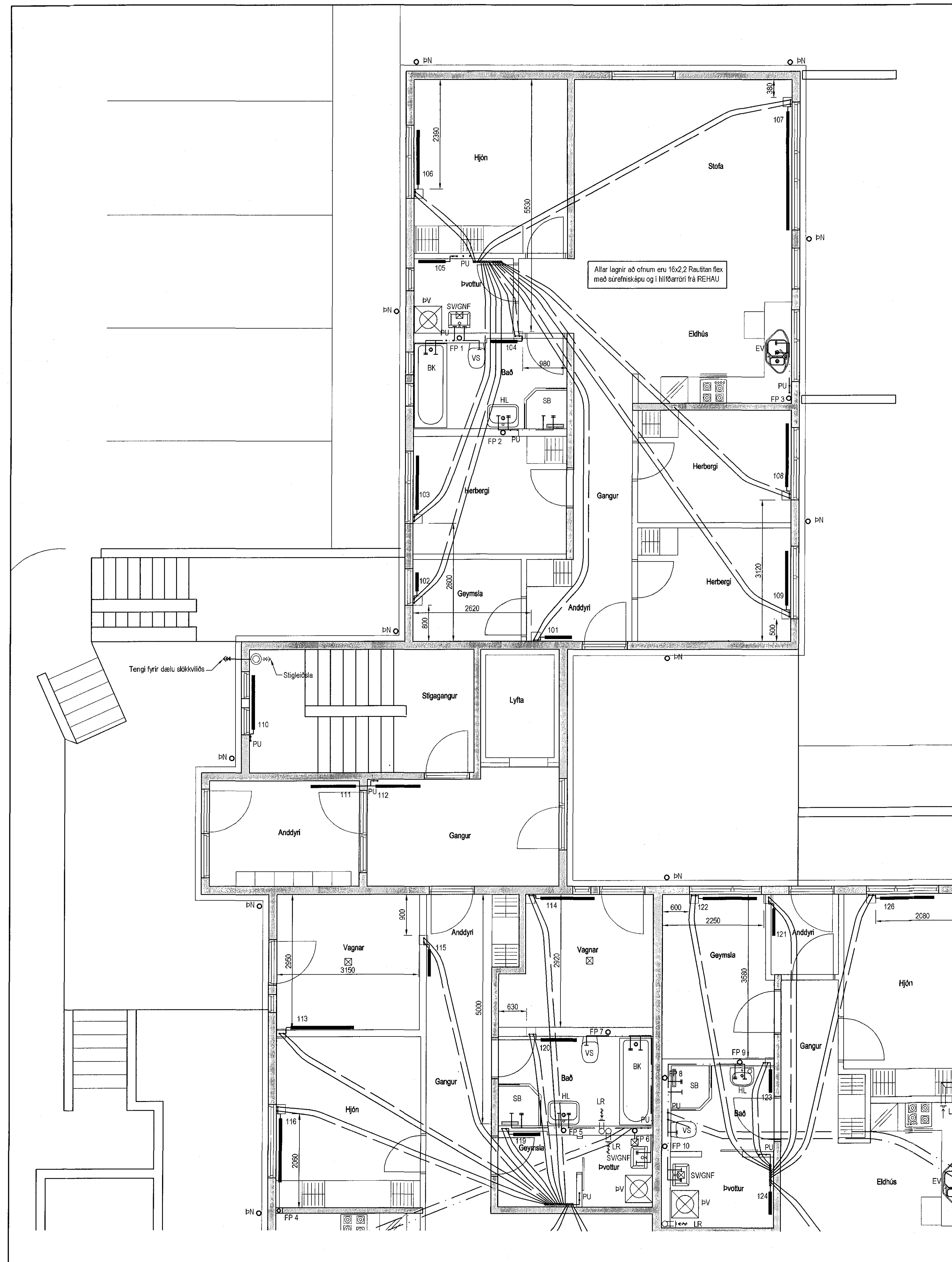
Lagnir 1. hæð, Grunnmynd 1:50
