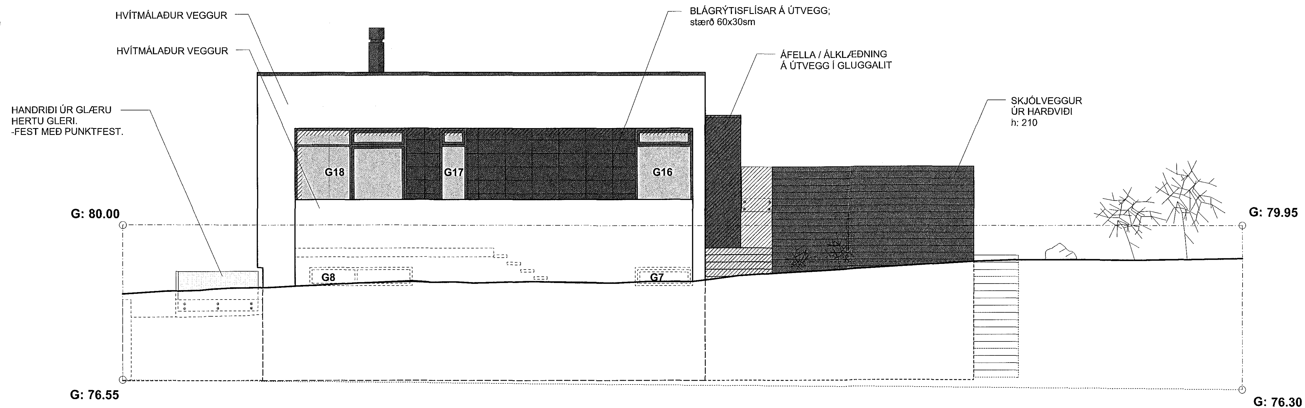
ÚTLIT VESTUR -með steypu handriði/vegg
