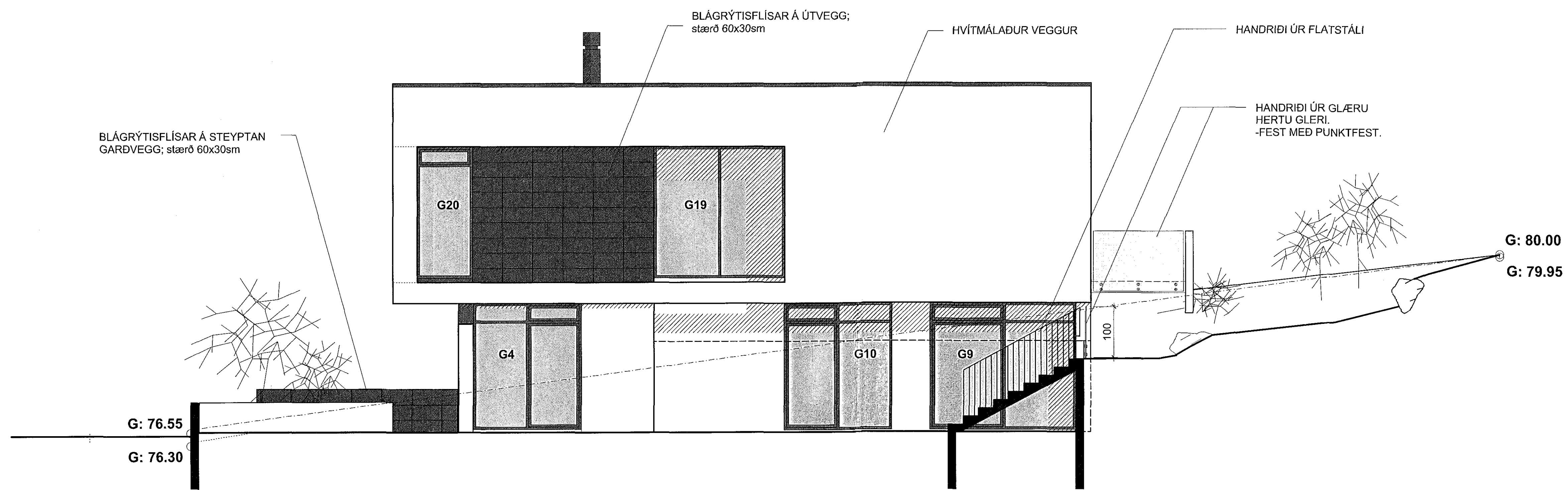
ÚTLIT NORÐUR -án stoð/skjólveggs
