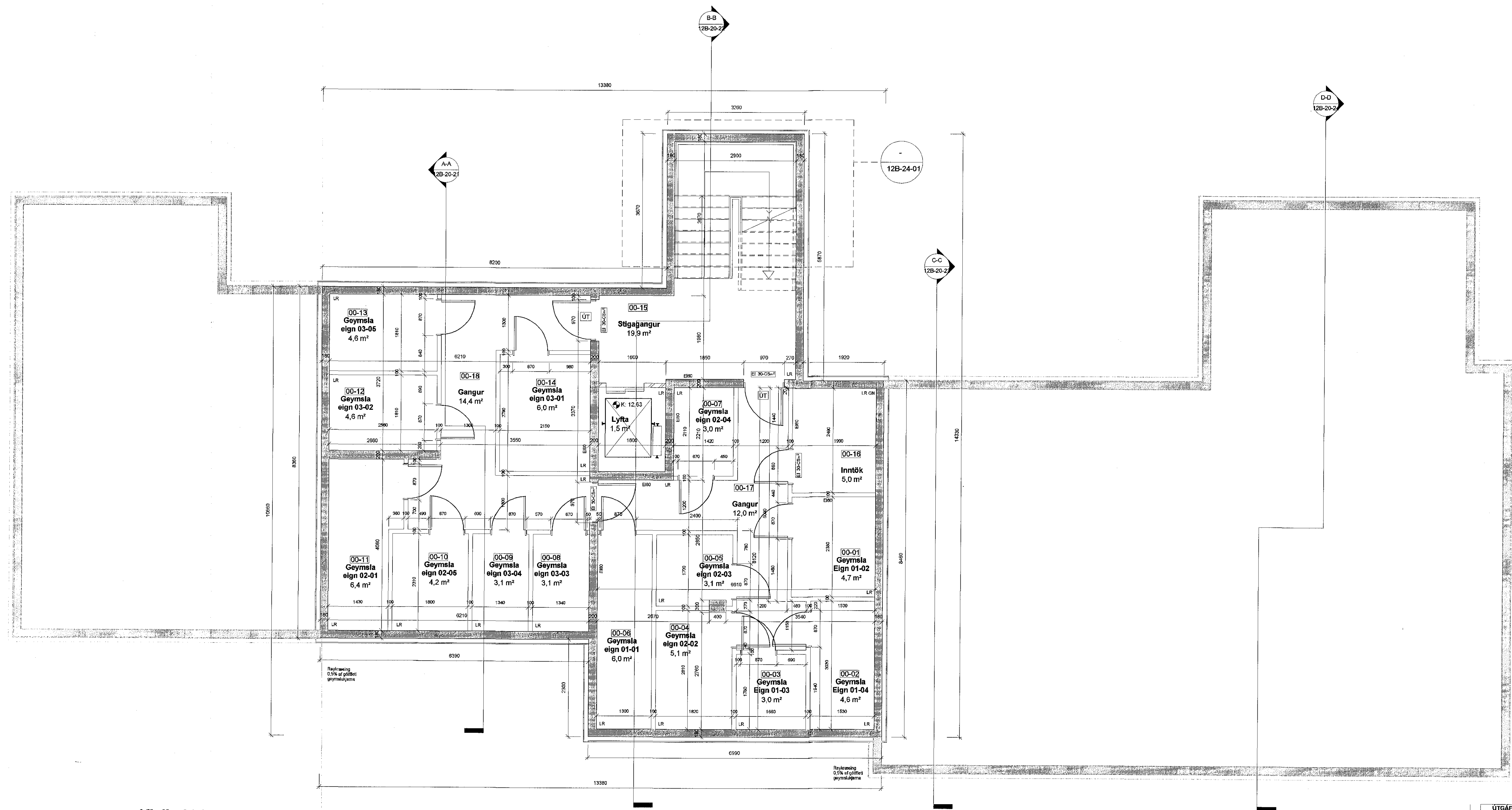
1 Kjallari 50 1 : 50
