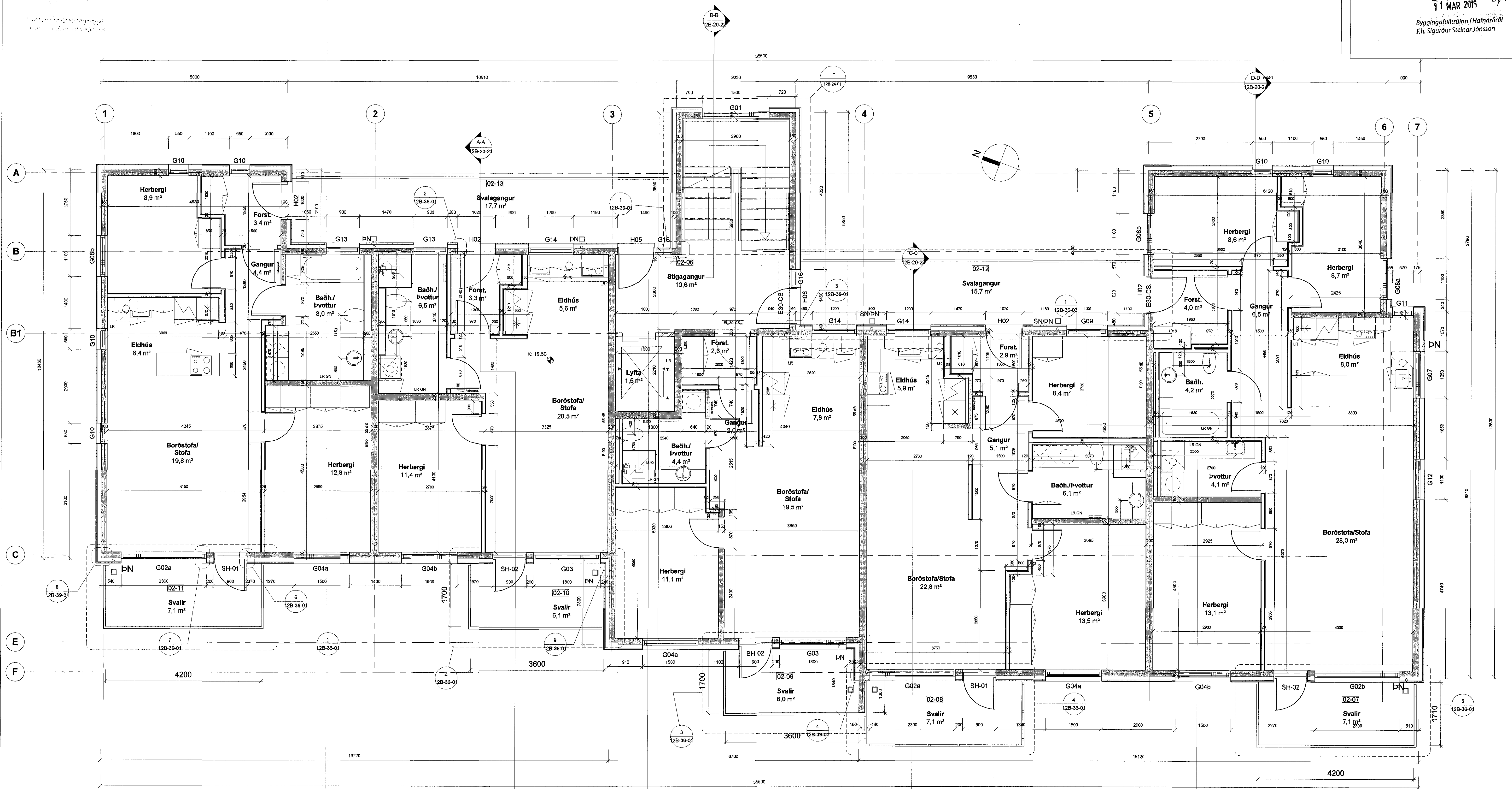
1 Hæð 2 50 1 : 50
