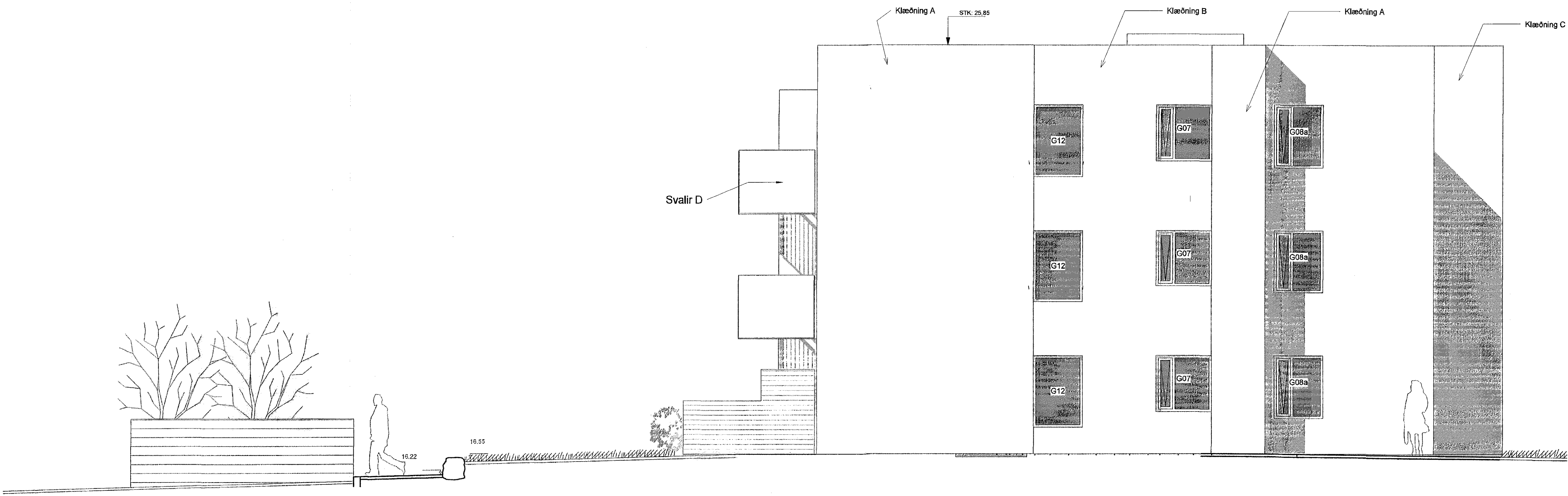
2 Suðurhlíð 1:50
