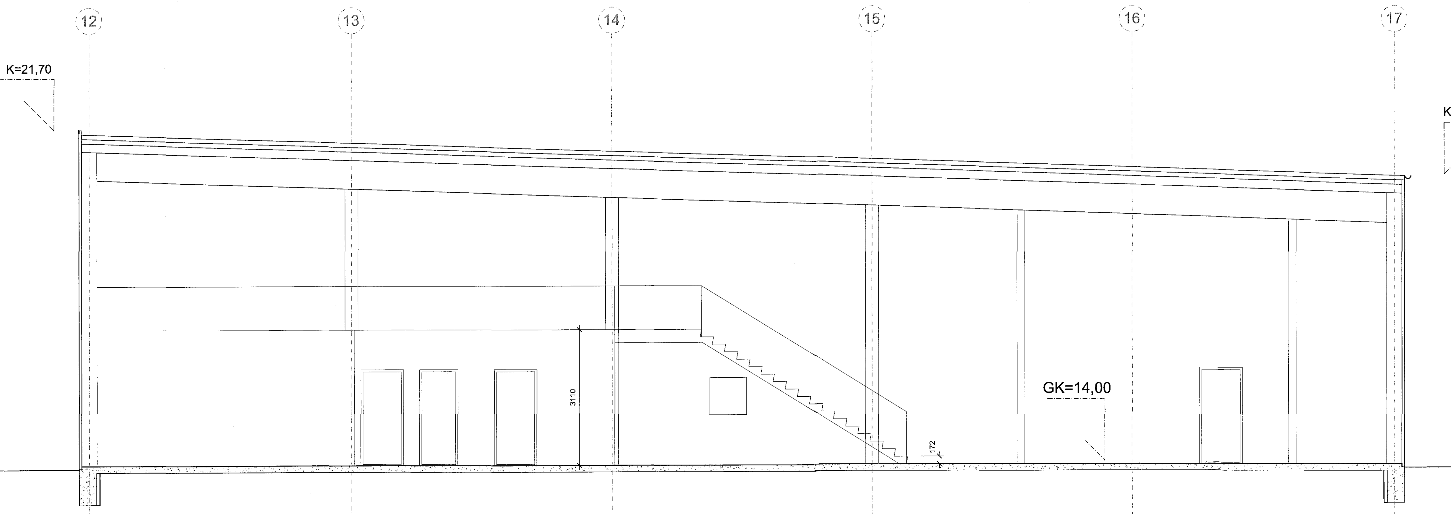
SNEIDING E-E, 1:50
