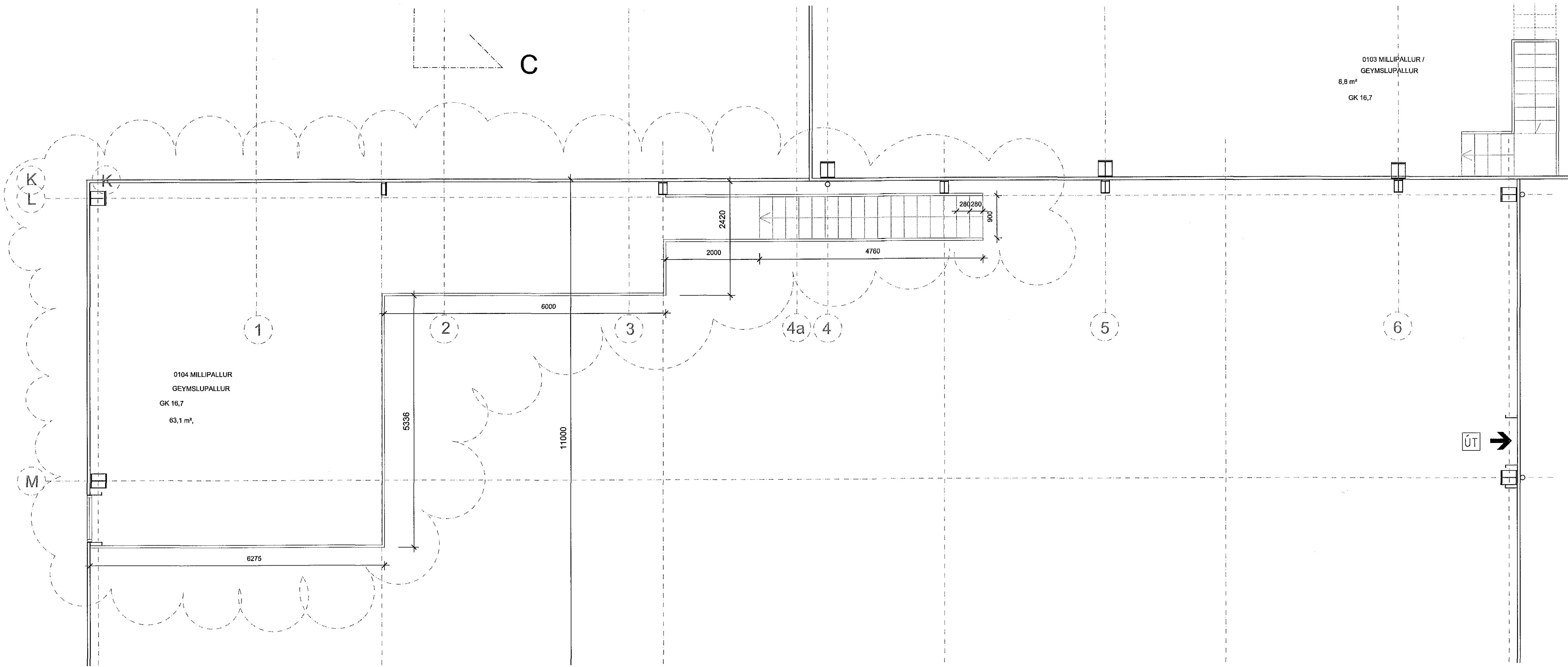
GRUNNMYND MILLIPALLUR Í VIÐBYGGINGU, 1:50
