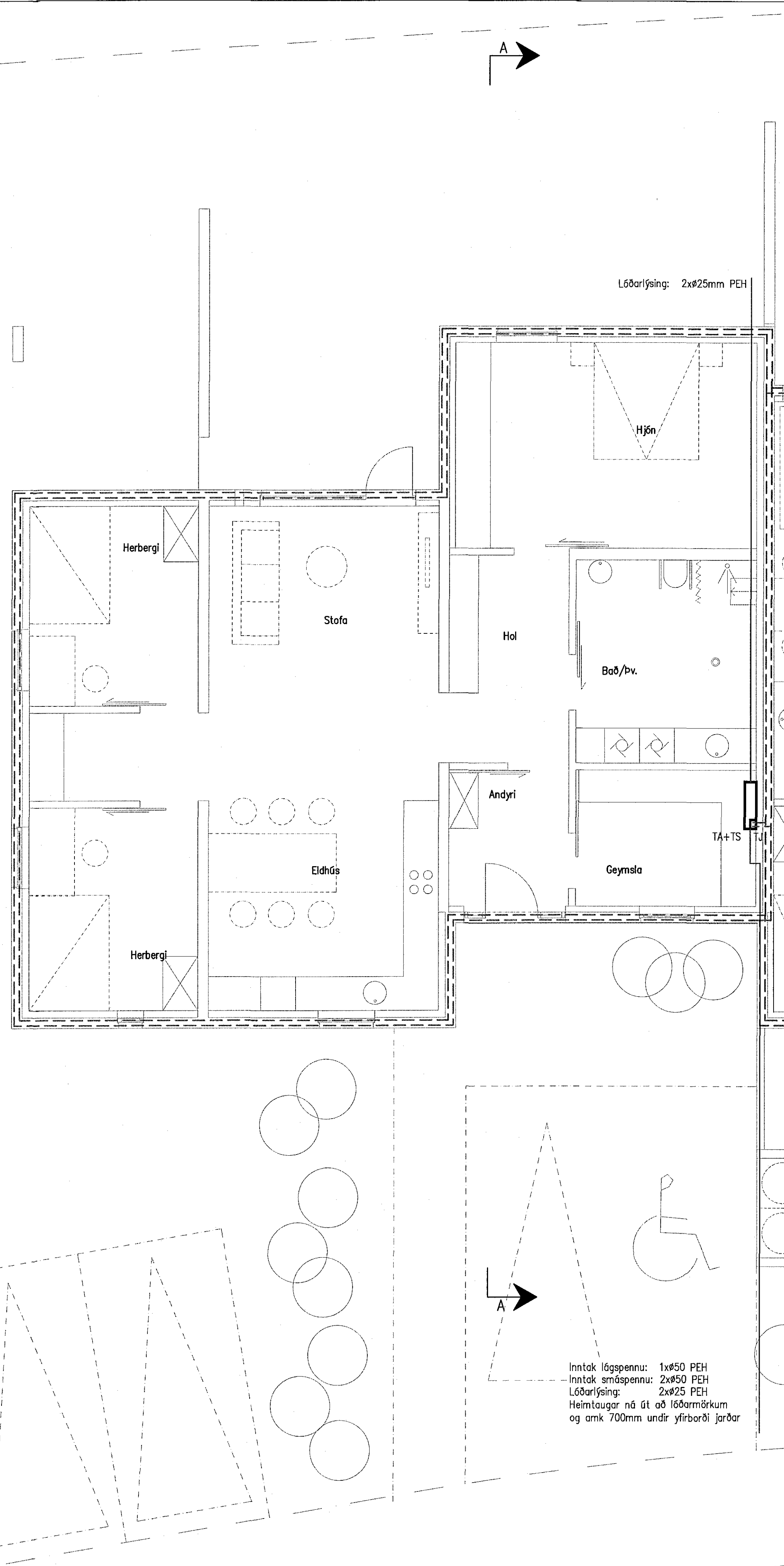
Sökkulskaut 1.hæð, 1:50
