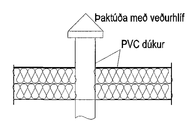
Snið í loftúður fyrir loftræstingu fallþípa 1:20
