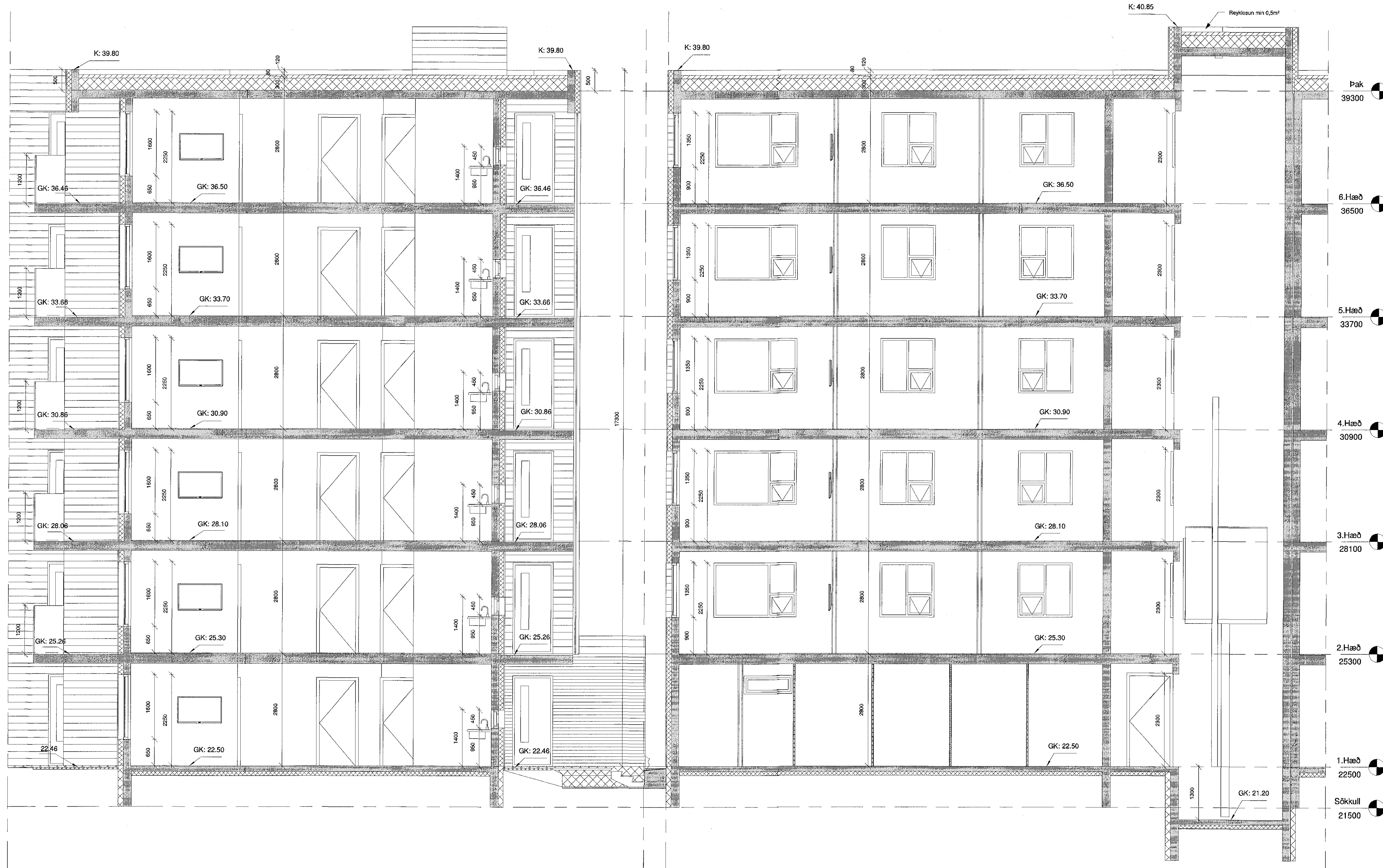
A A Snið 1 : 50
