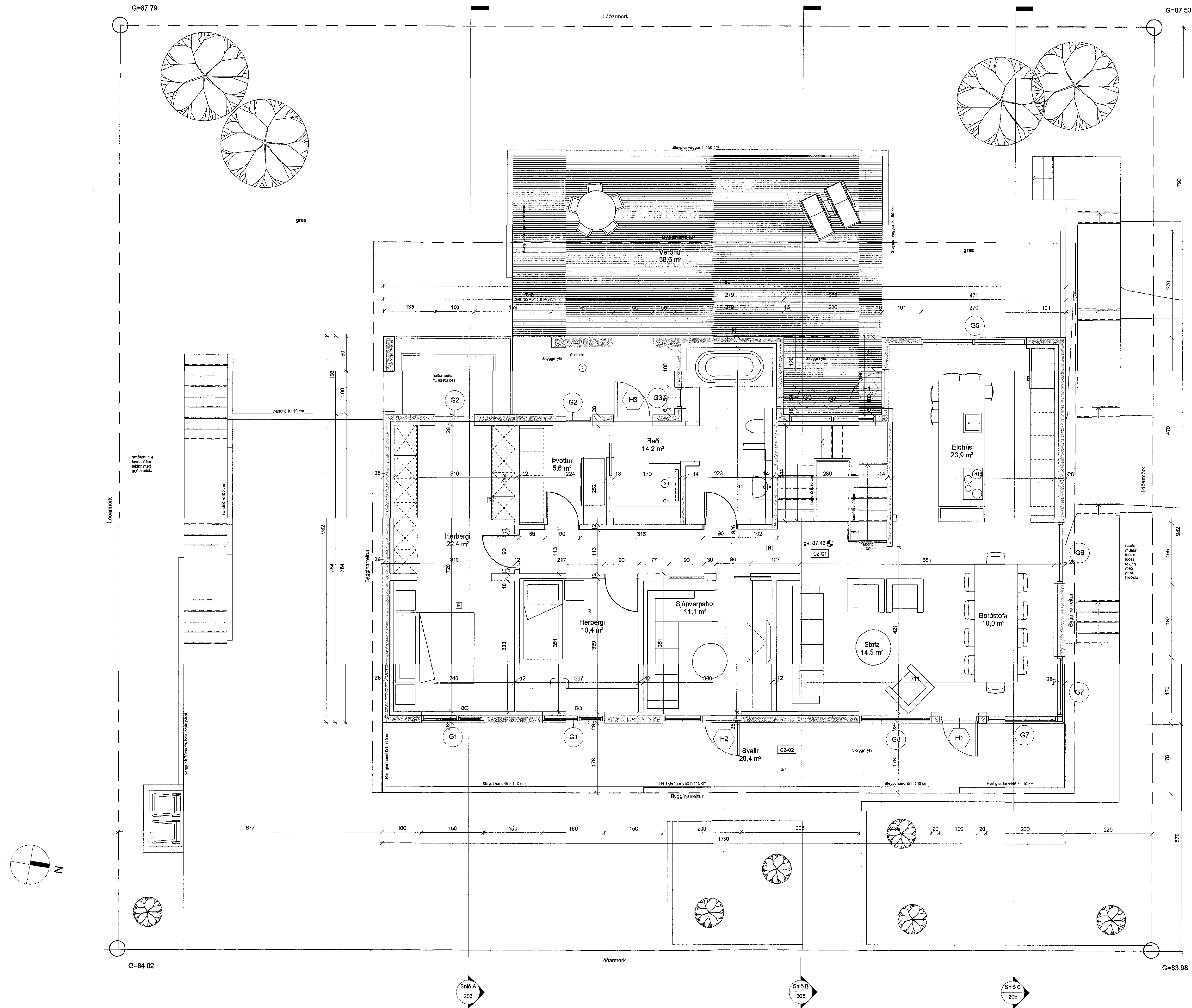
Hæð 2 sérteikning 1 : 50
