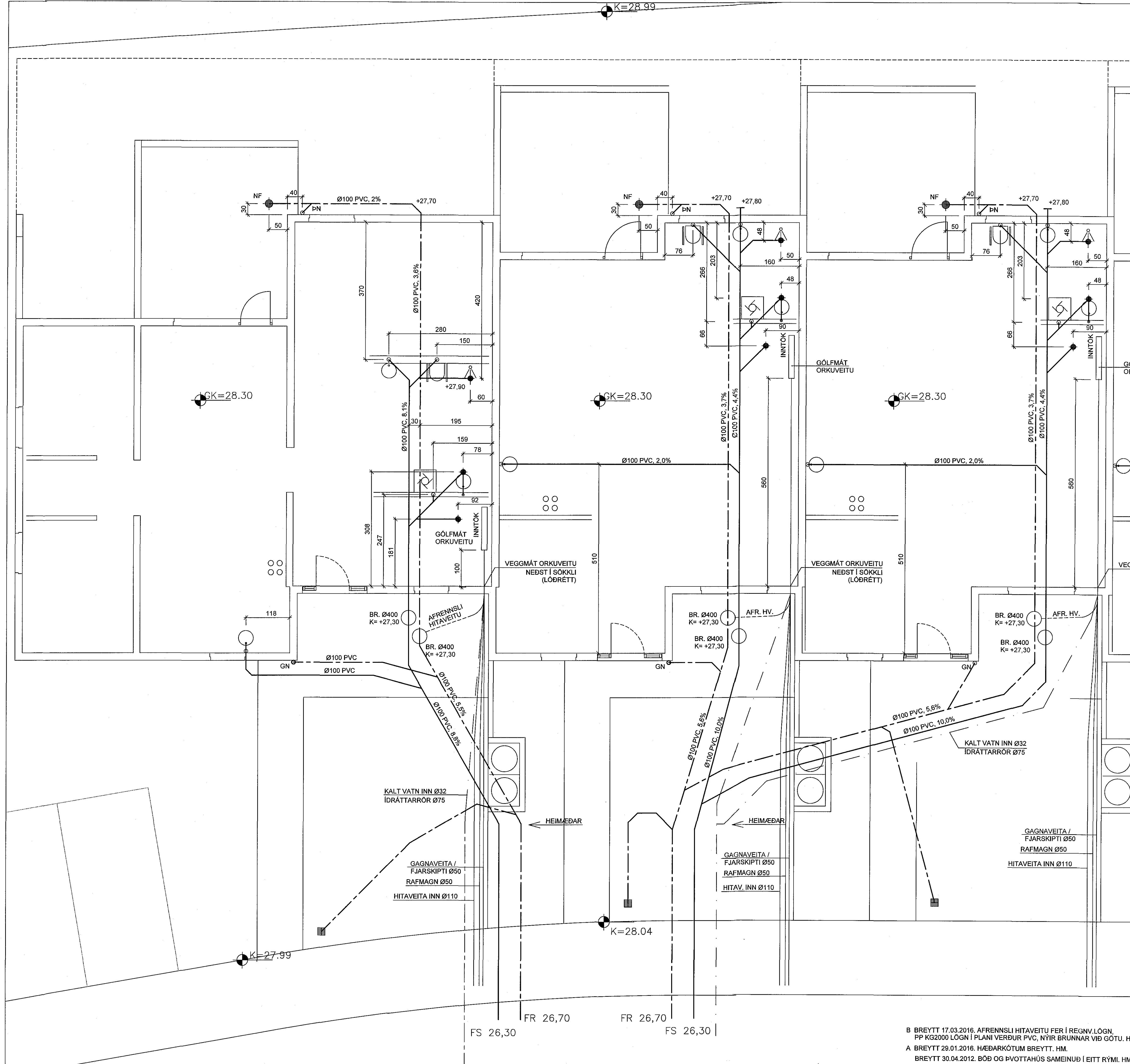
AFSTÖÐUMYND, 1:500
