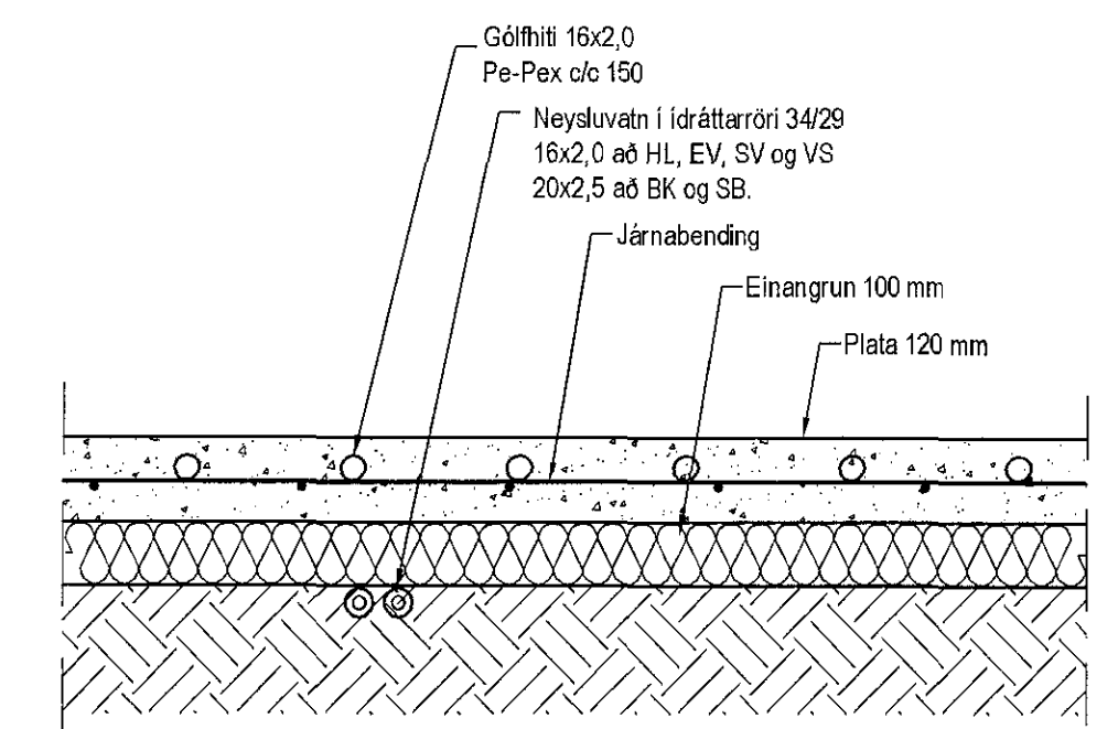
Hita- og vatnslagnir, Snúð í botnplötu, 1:10
