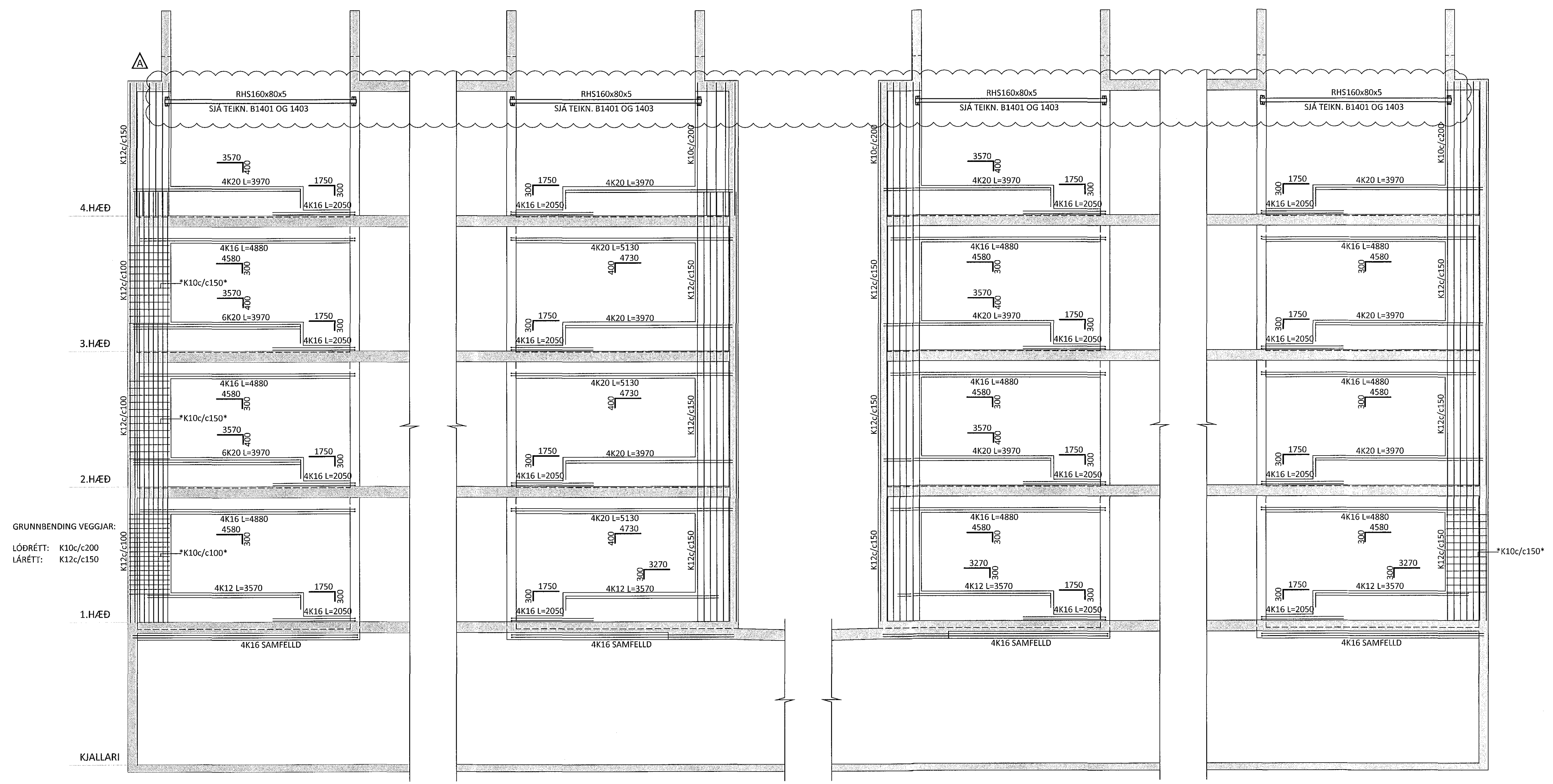
V056b M1:50
