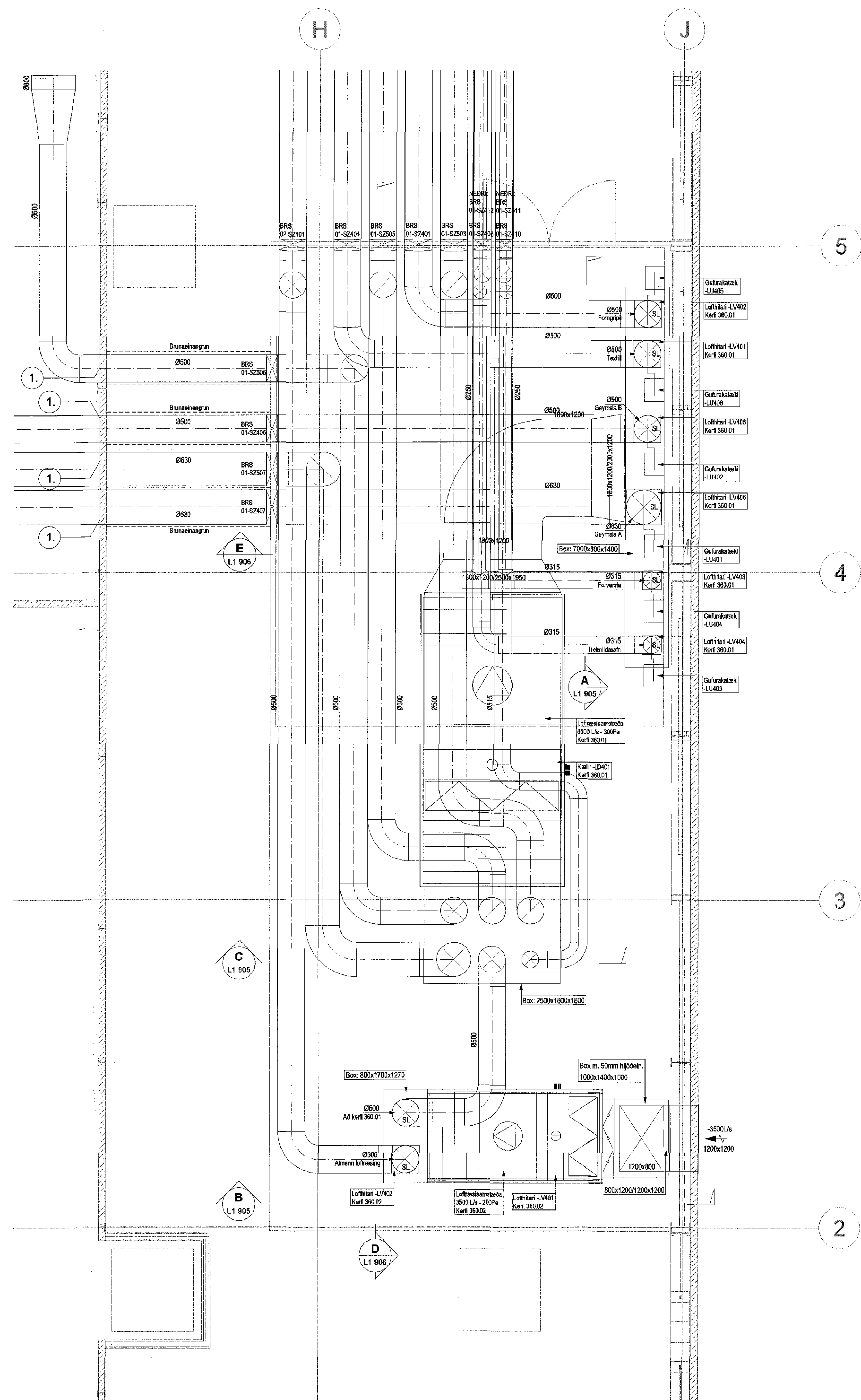
② Grunnmynd loftræsikerfis - við þak Mkv. 1:20
