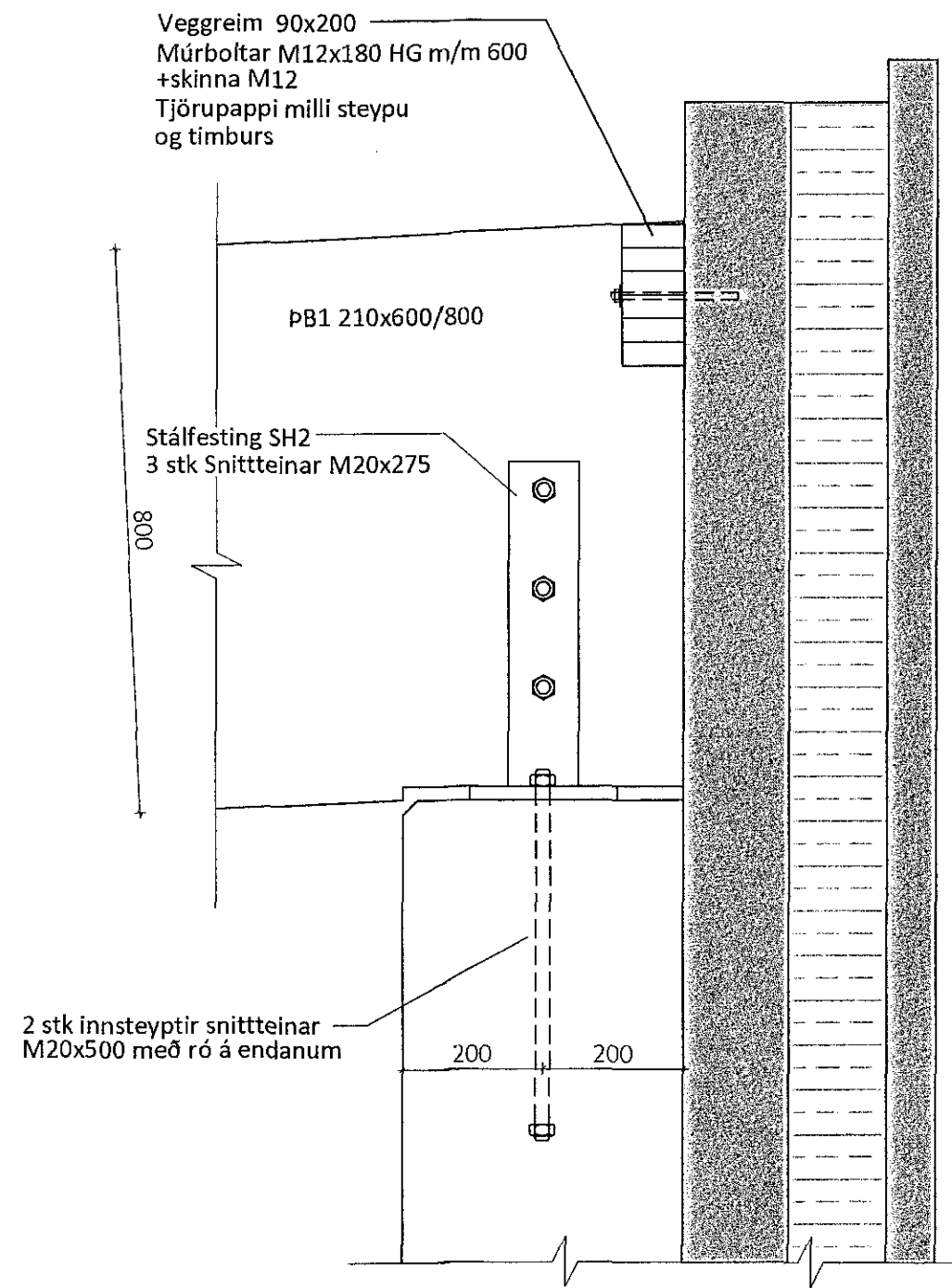
Sérmynd 2 Mkv.: 1:10 302
