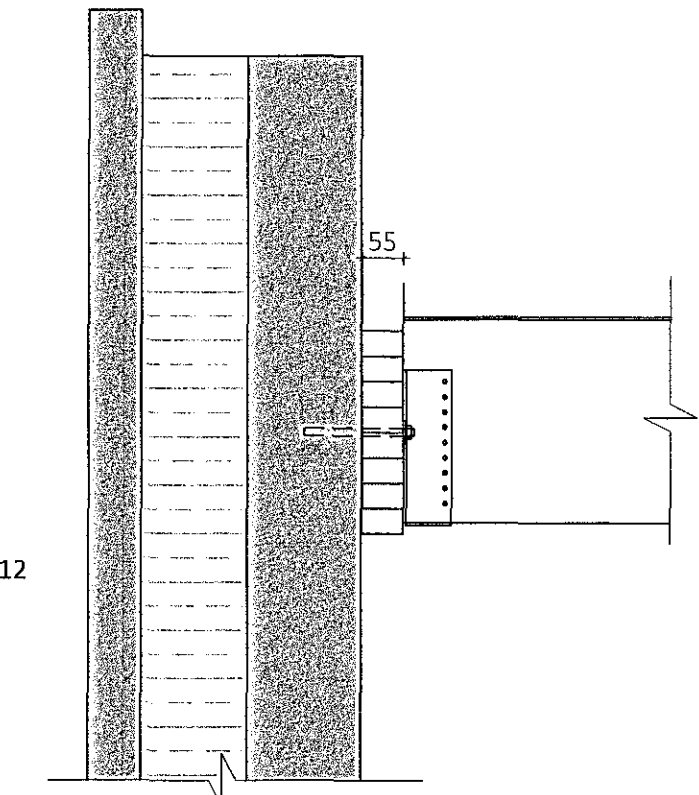
Snið A-A
