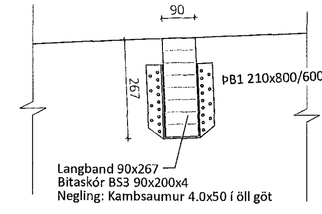
Sérmynd 3 Mkv.: 1:10 302
