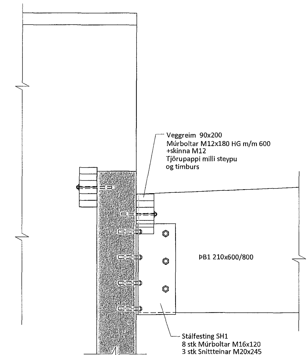
Snið A-A
