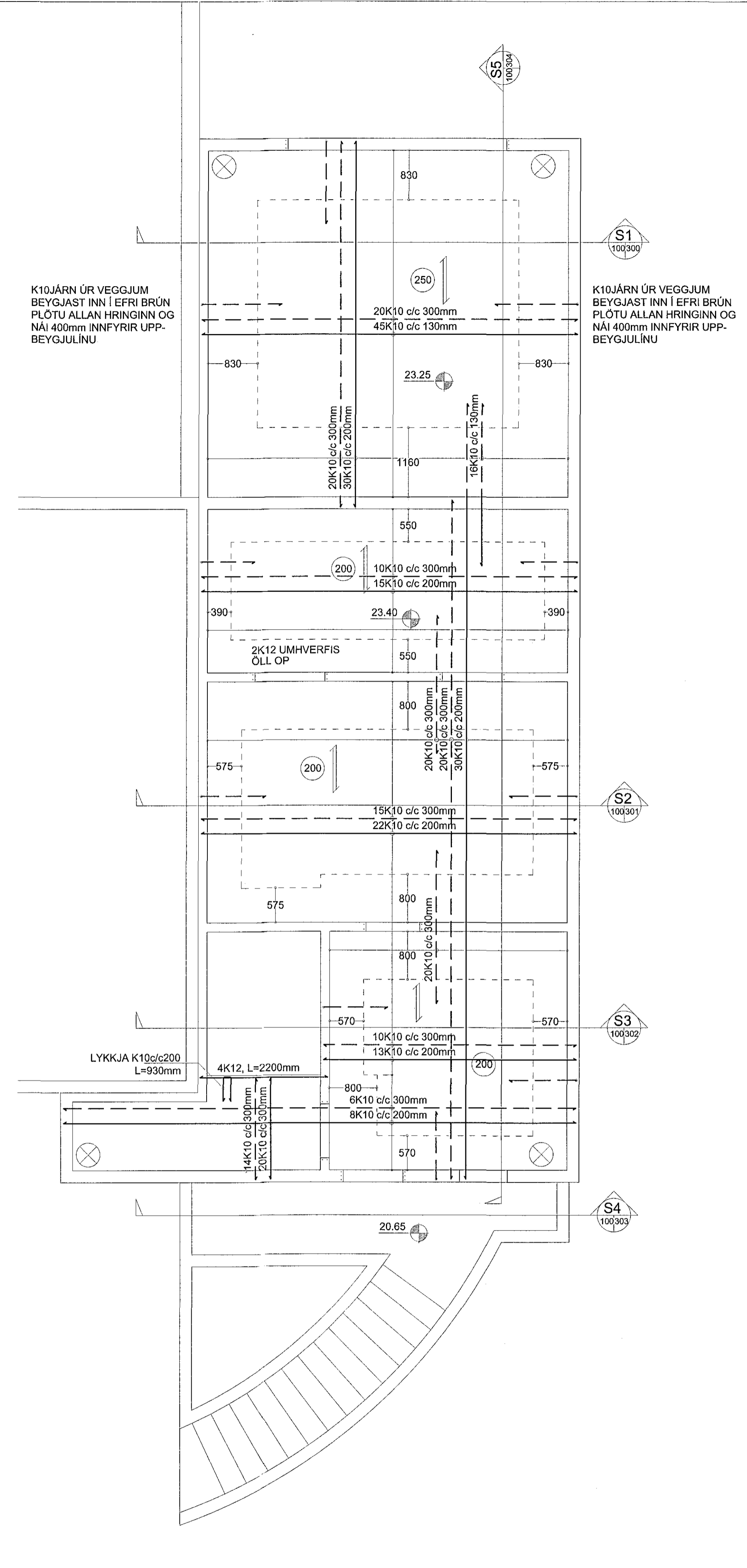
JARDHÆÐ mkv. 1:50
