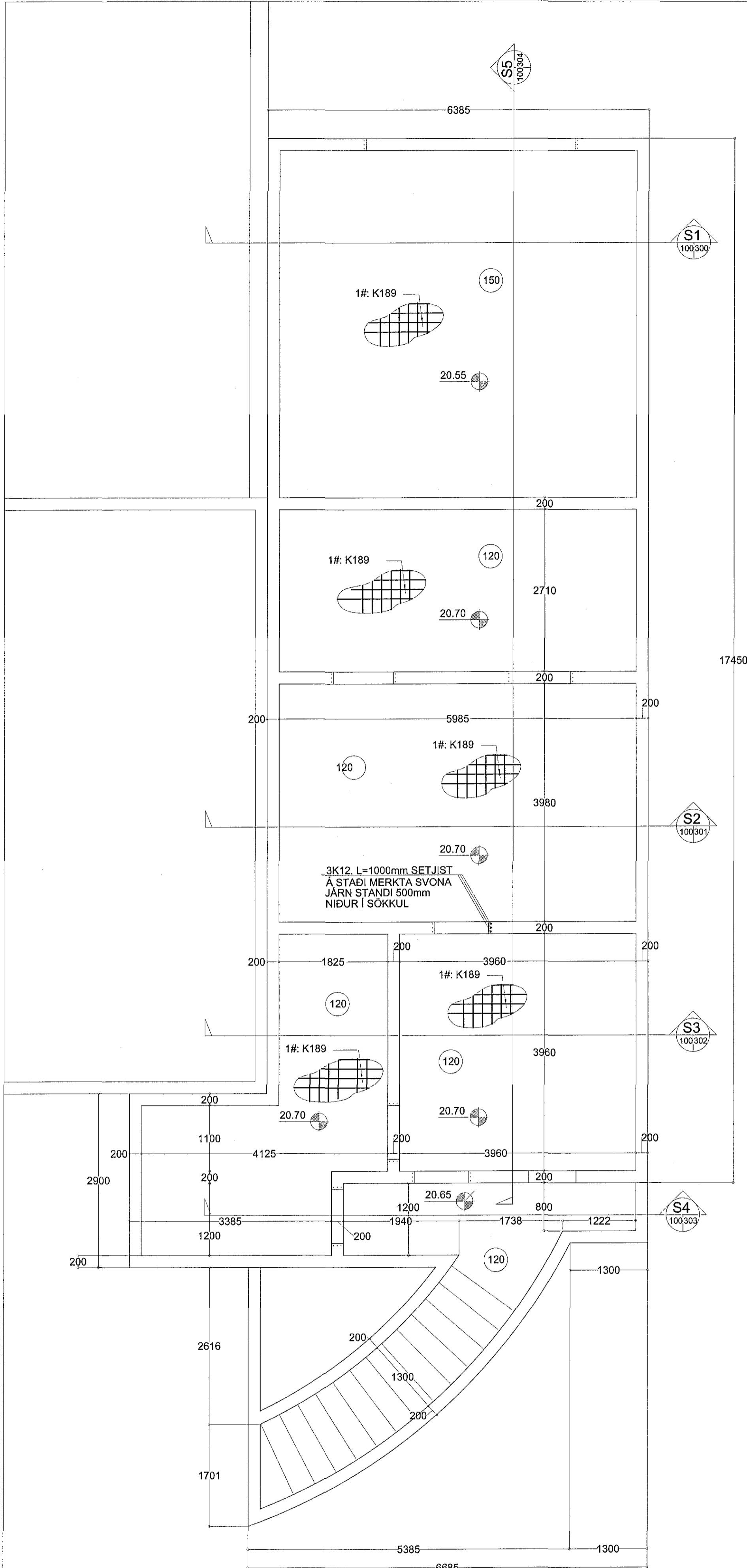
SÖKKULL mkv. 1:50
