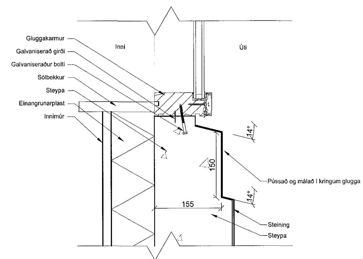
ÚRTAK KRINGUM GLUGGA LÓÐRÉTT SNIÐ
