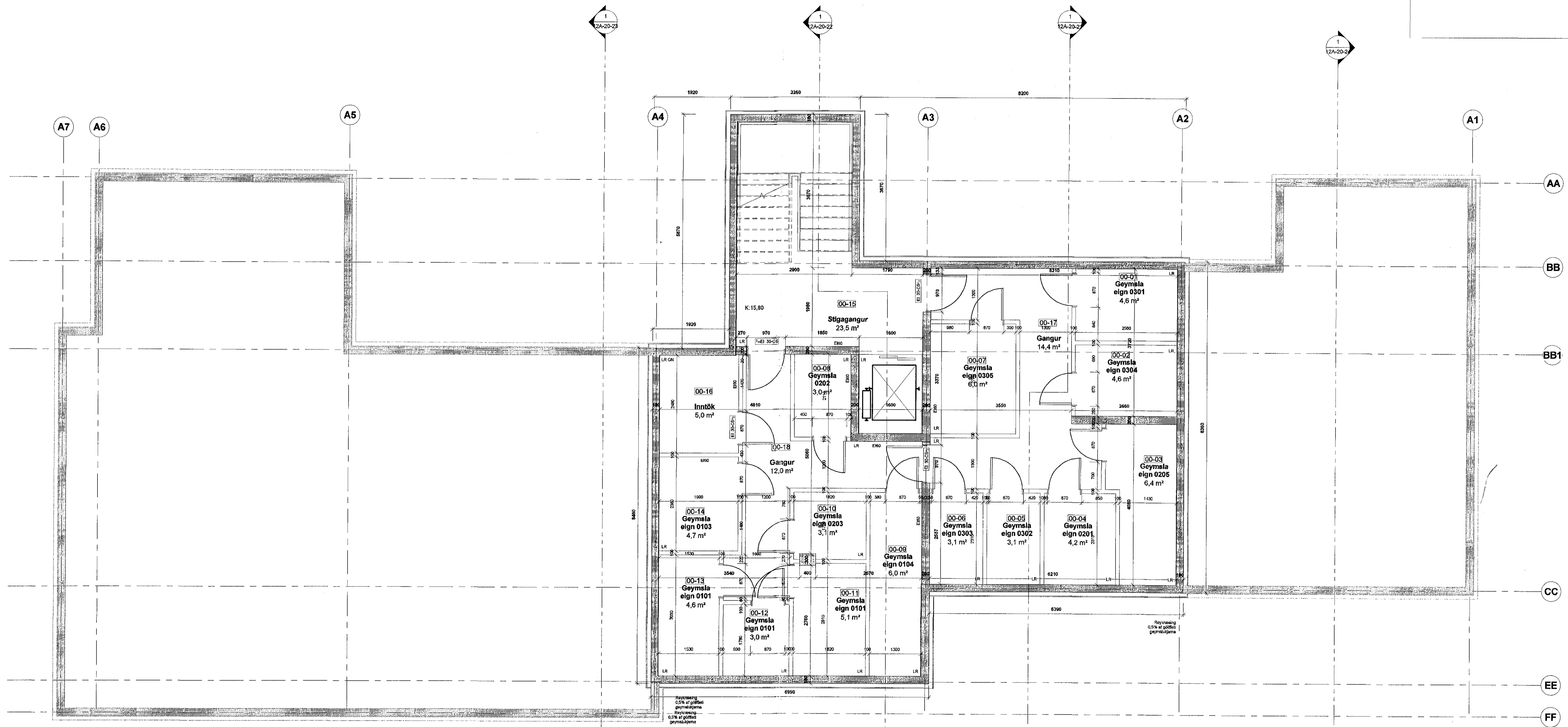
1 Kjallari 50 - 12A 1 : 50
