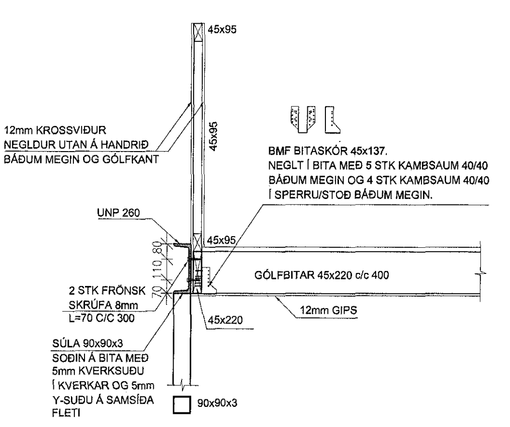
2 SNID B100,101 M. 1: 20
