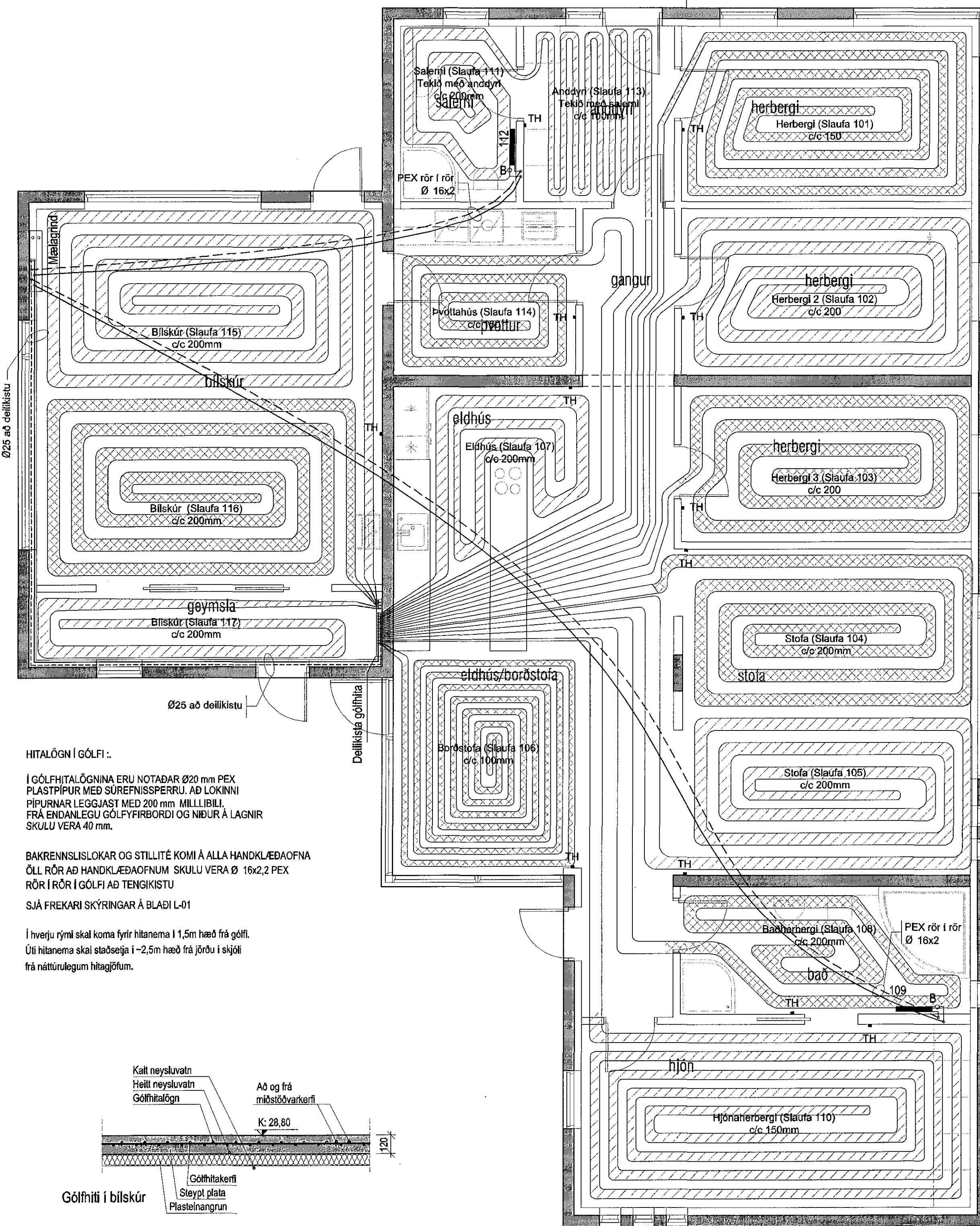
Grunnmynd miðstöðvarlagna 1:50
