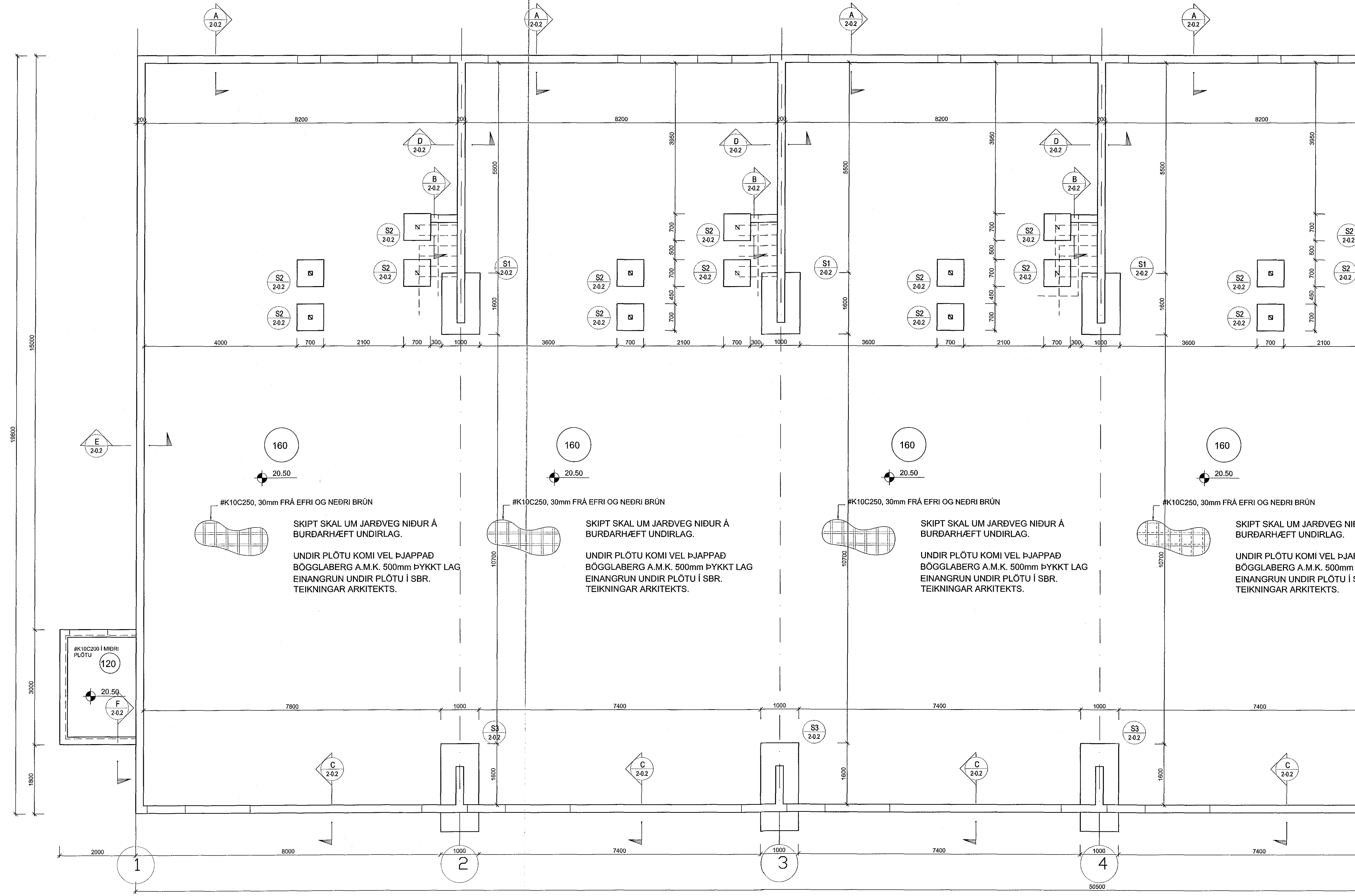
GRUNNMYND SÖKKLA, 1:50
