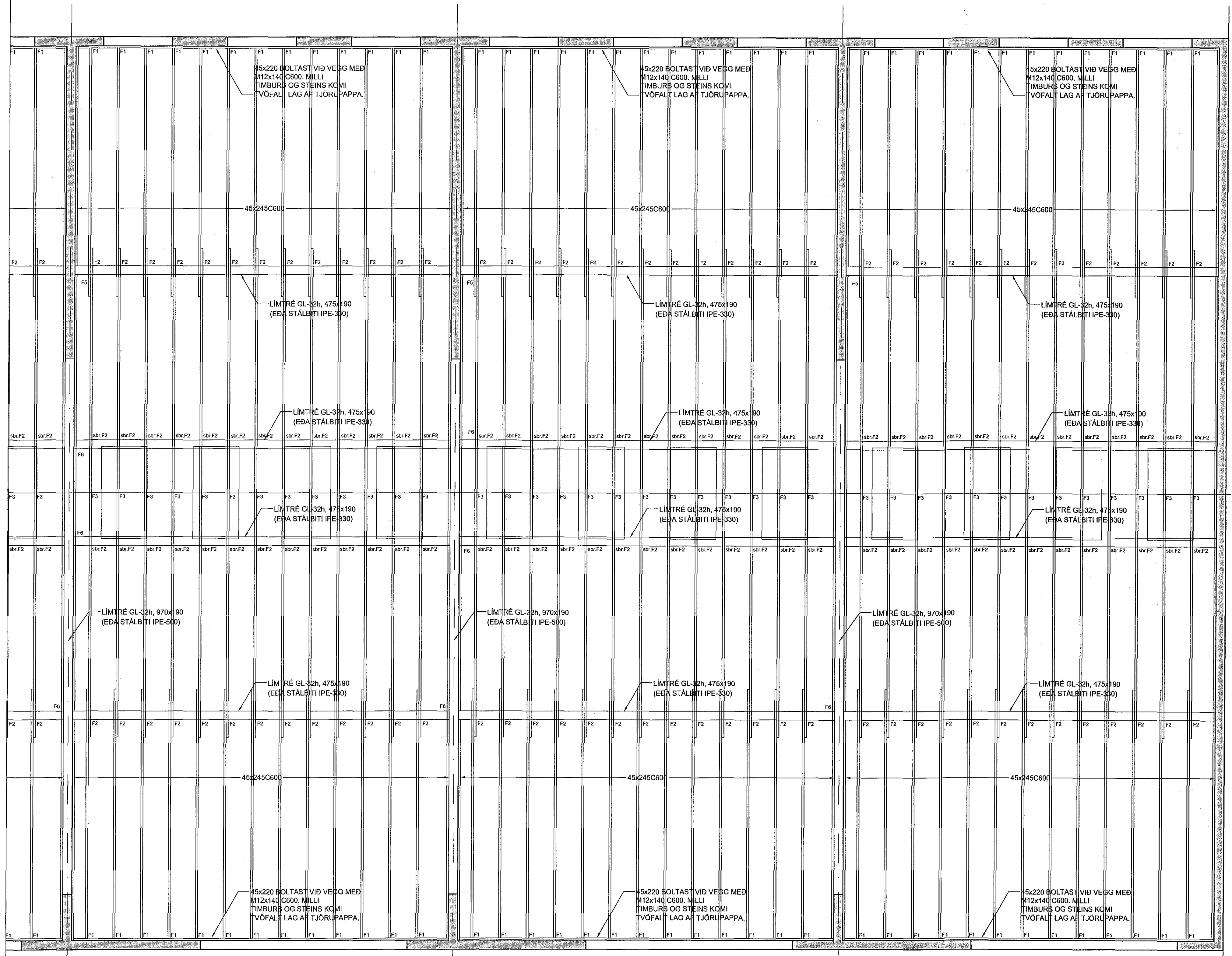
GRUNNMYND ÞAKS, 1:50
